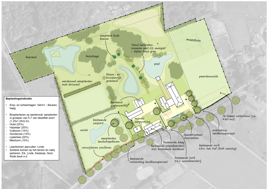
Figuur 3: Tekening van de toekomstige situatie
