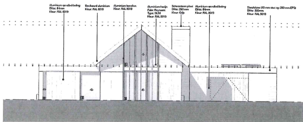
VOORAANZICHT
