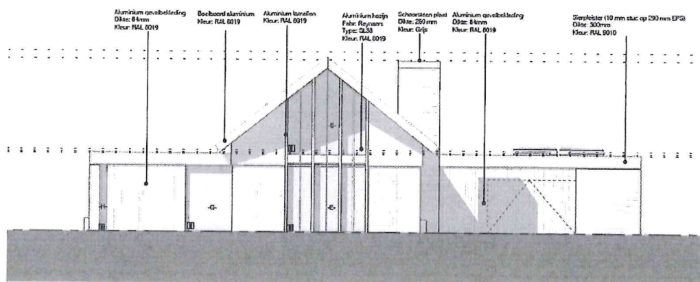
VOORAANZICHT
