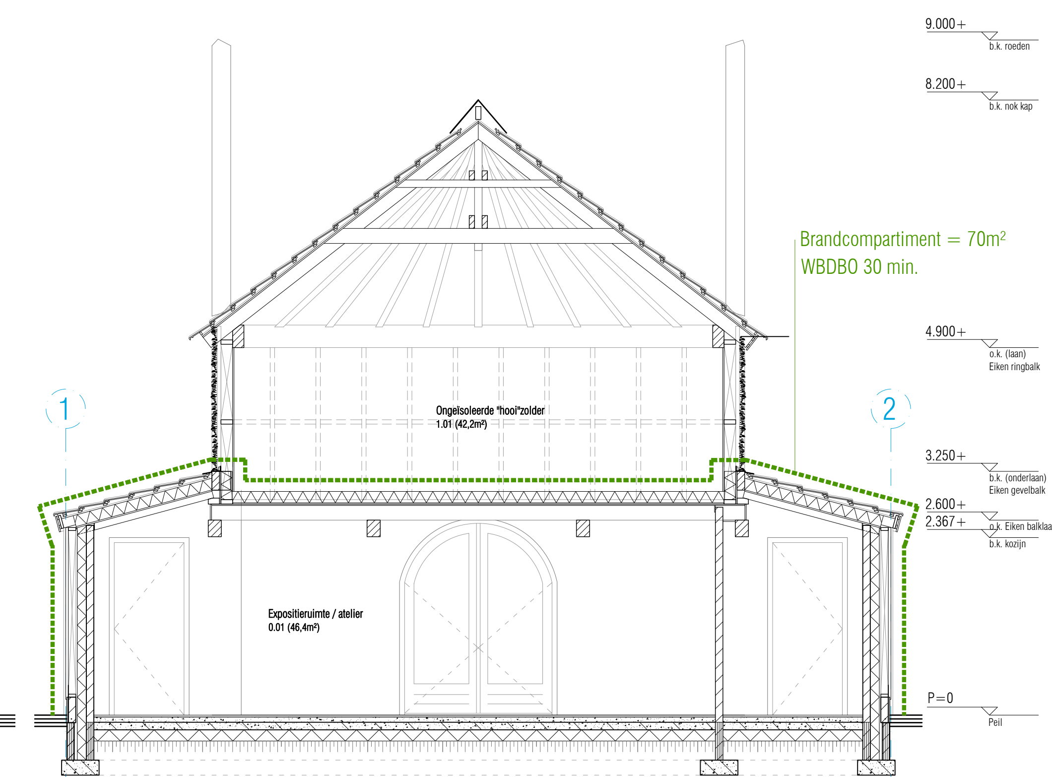
DOORSNEDE A
