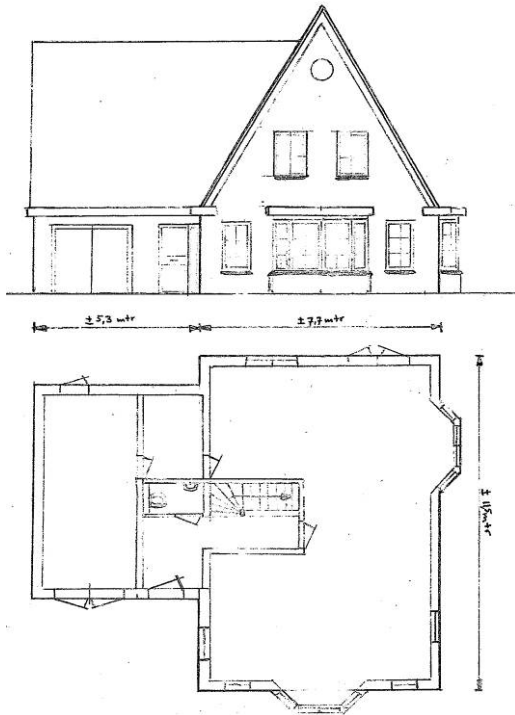
afbeelding 6: voorlopig ontwerp
