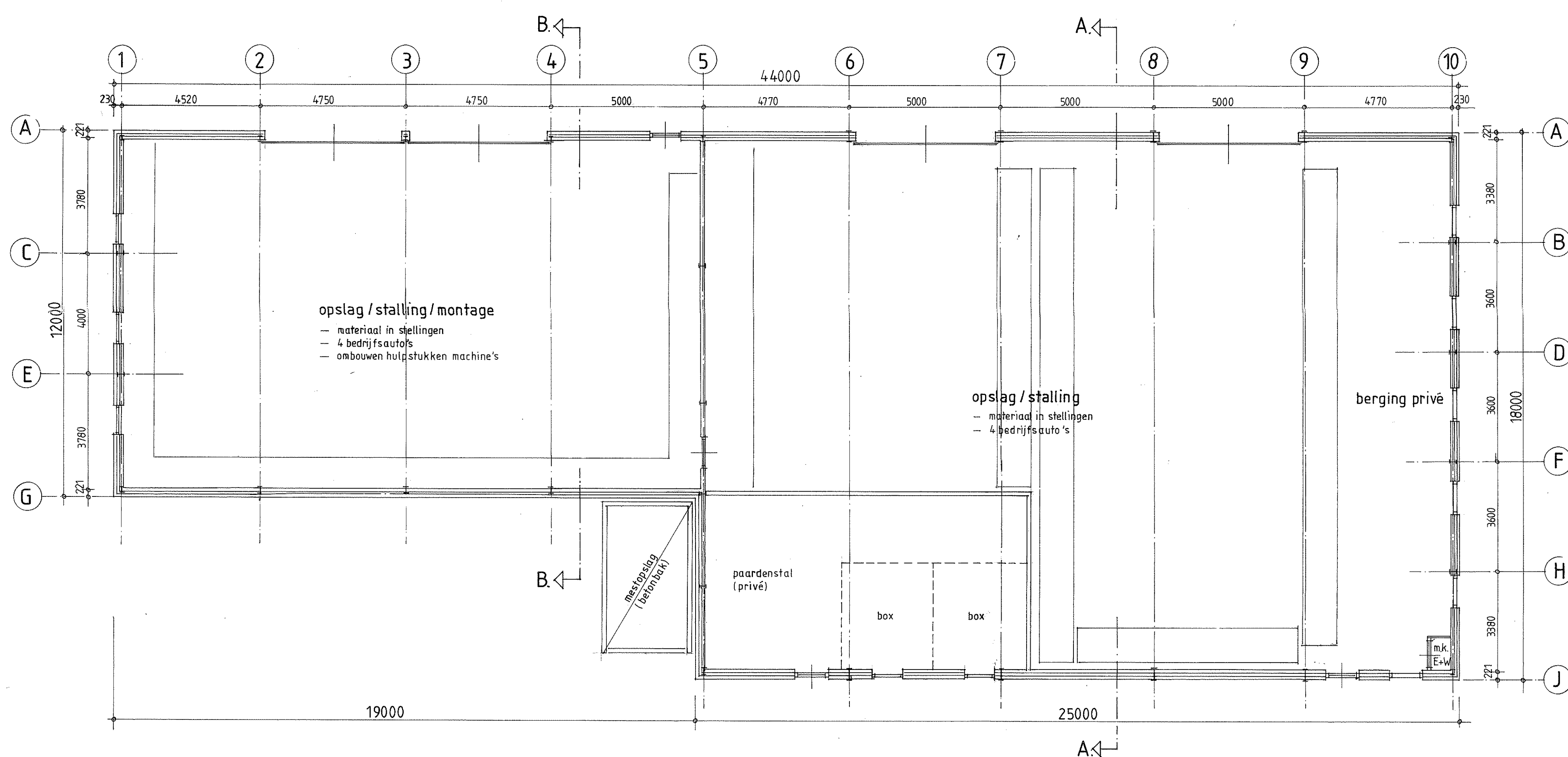
Plattegrond
