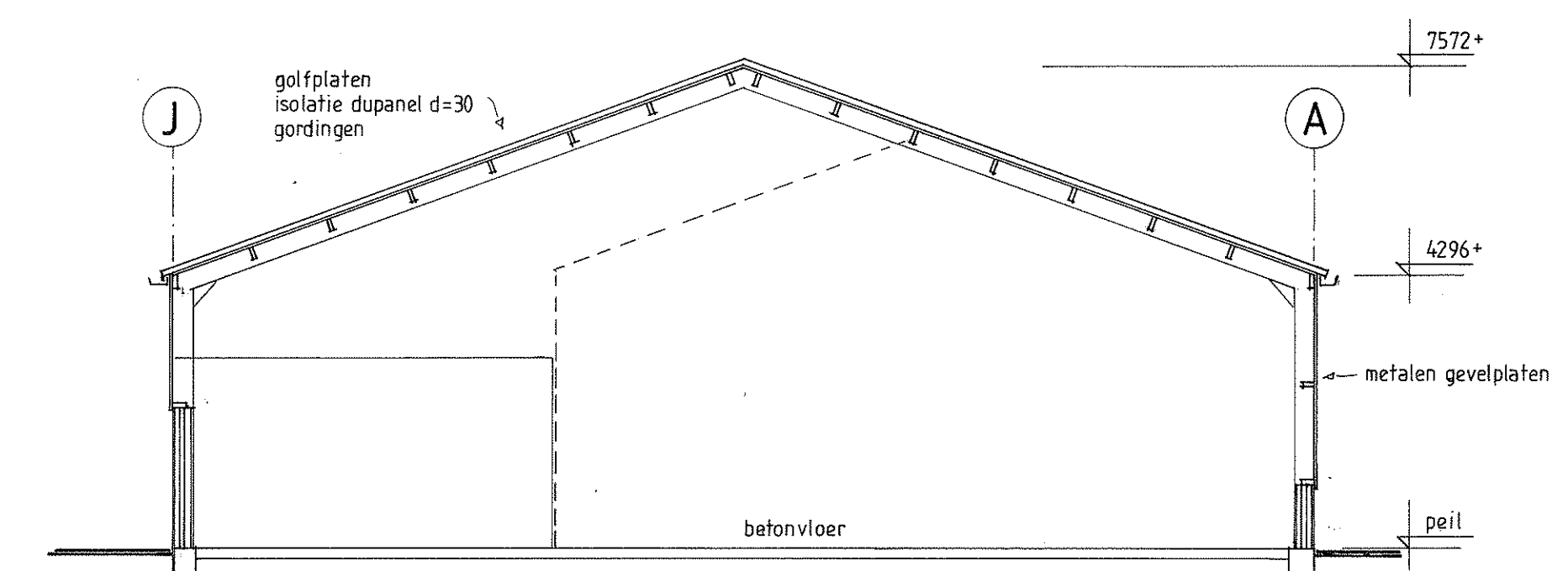
Doorsnede A-A
