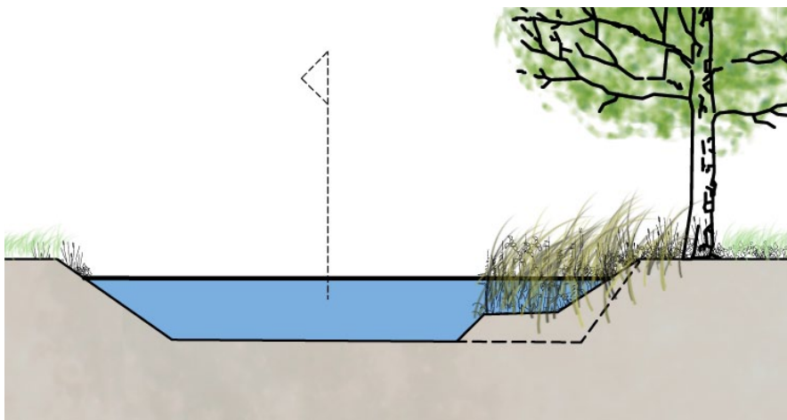
principe natuurvriendelijke oever met plasberm
