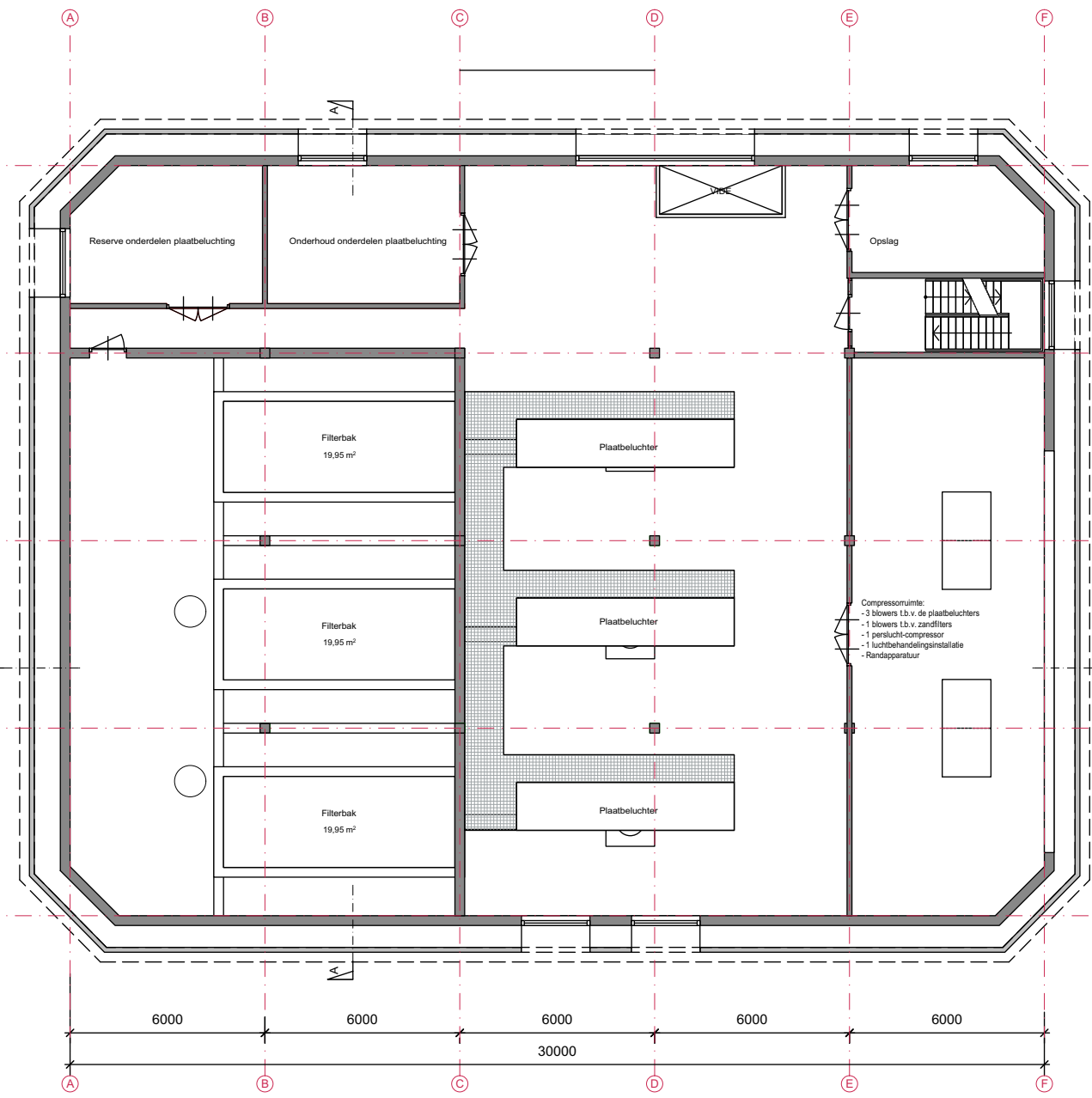
Verdieppingsvloer
