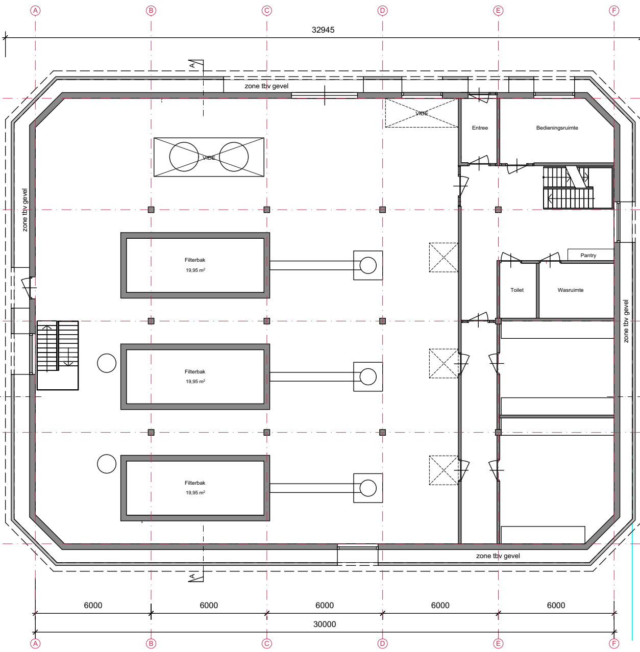
Begane grondvloer
