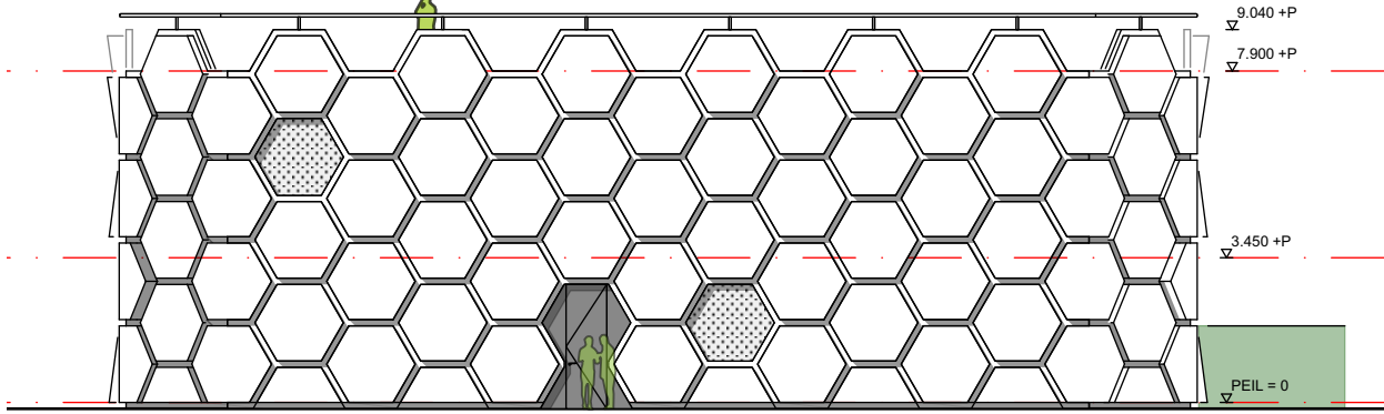
Westgevel
