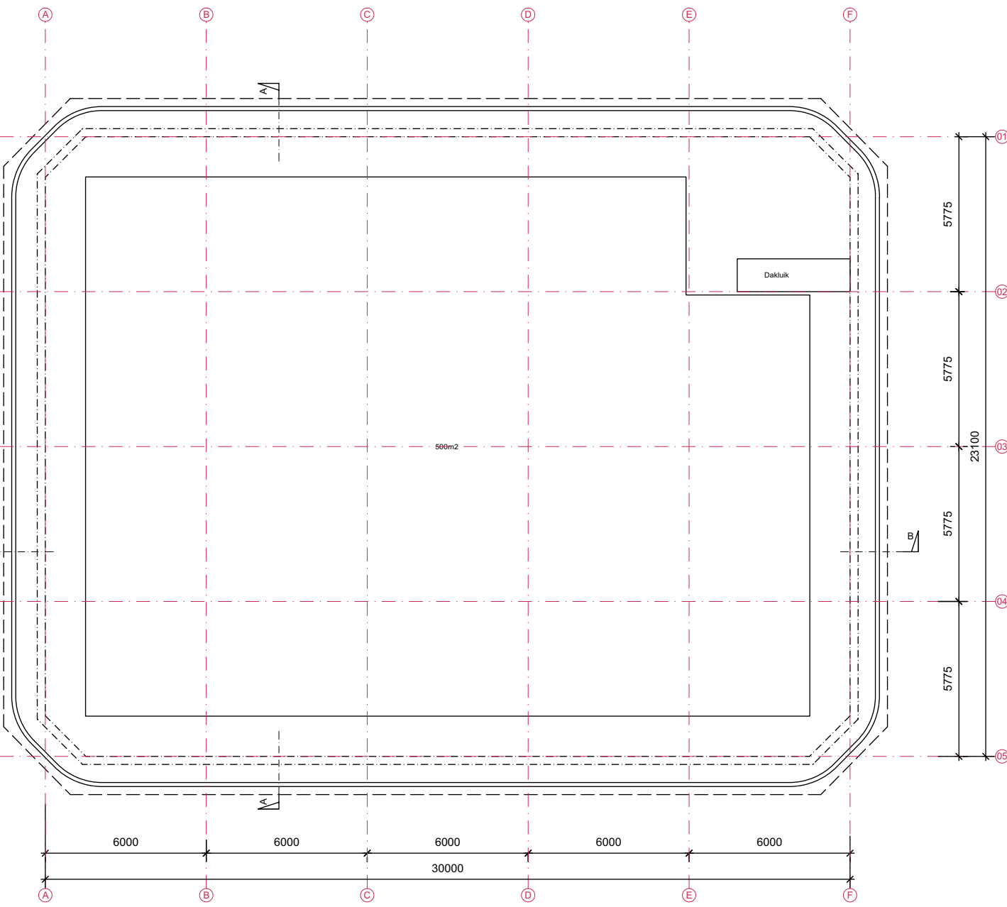
Dakvloer
