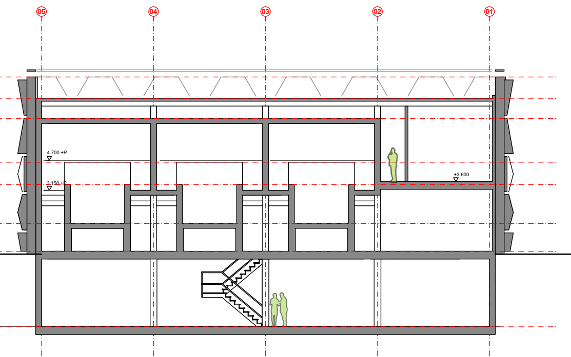
Dwarsdoorsnede AA
