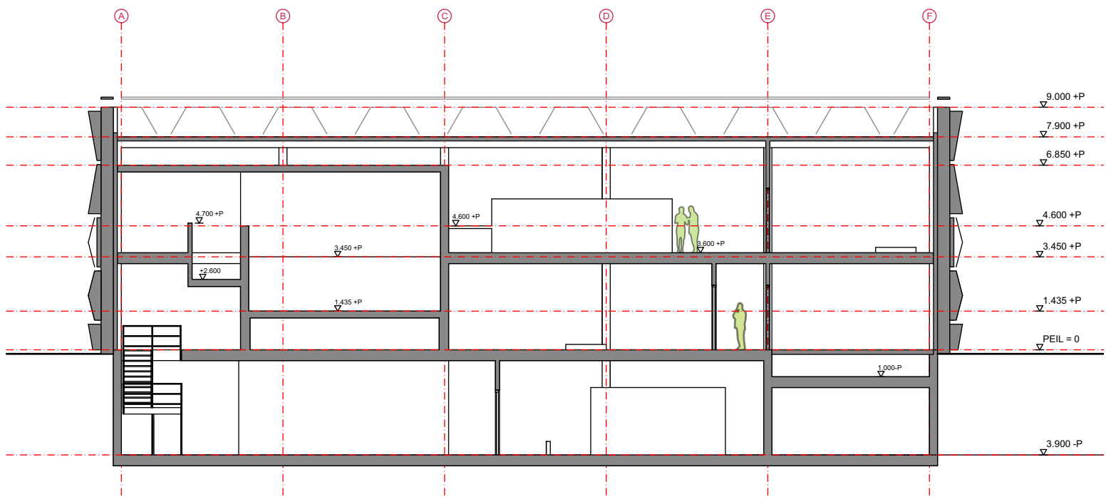
Langsdoorsnede BB
