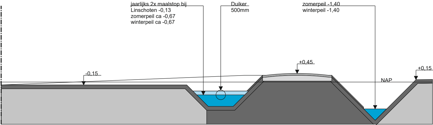
Doorsnede
