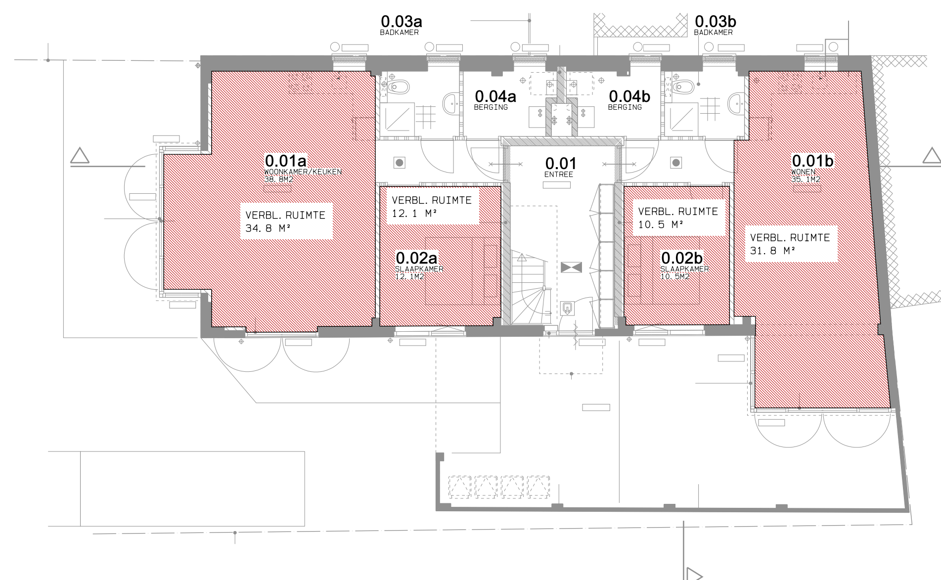
BEGANE GROND VERBLIJFSRUIMTEN
