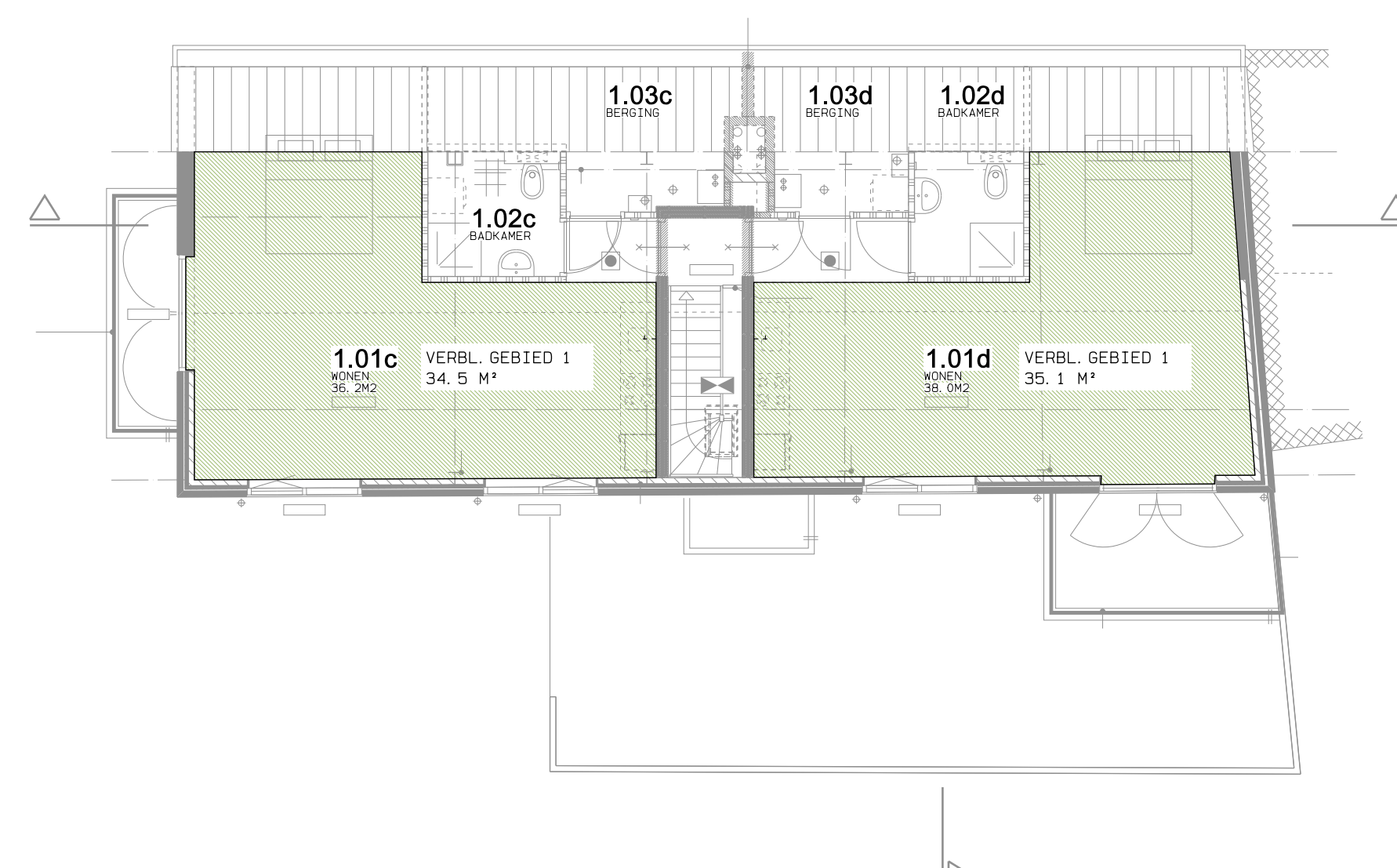
1 e VERDIEPING VERBLIJFSGEBIEDEN
