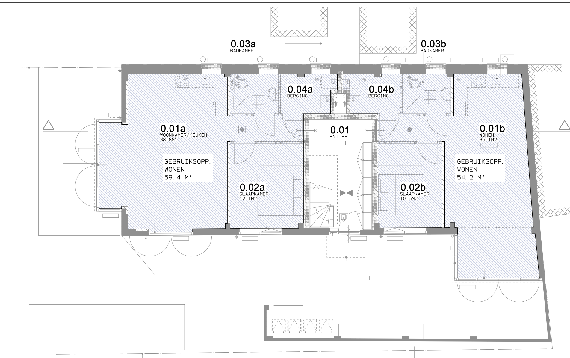
BEGANE GROND GEBRUIKSOPPERVLAKTE
