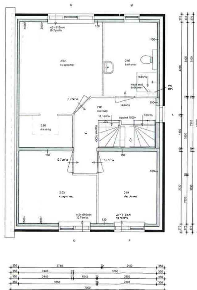
eerste verdieping
