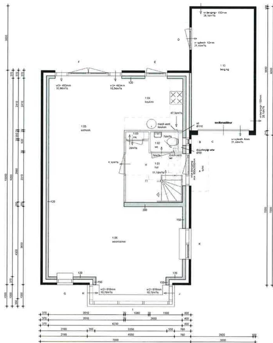
begane grond
