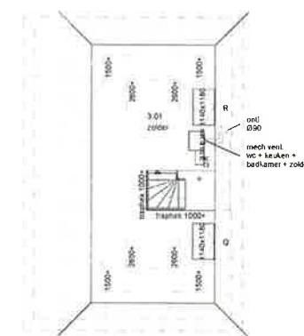
tweede verdieping
