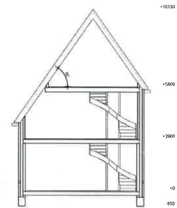
doorsnede
