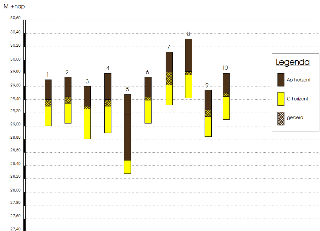
Figuur 18B: Boorprofielen 1-10
