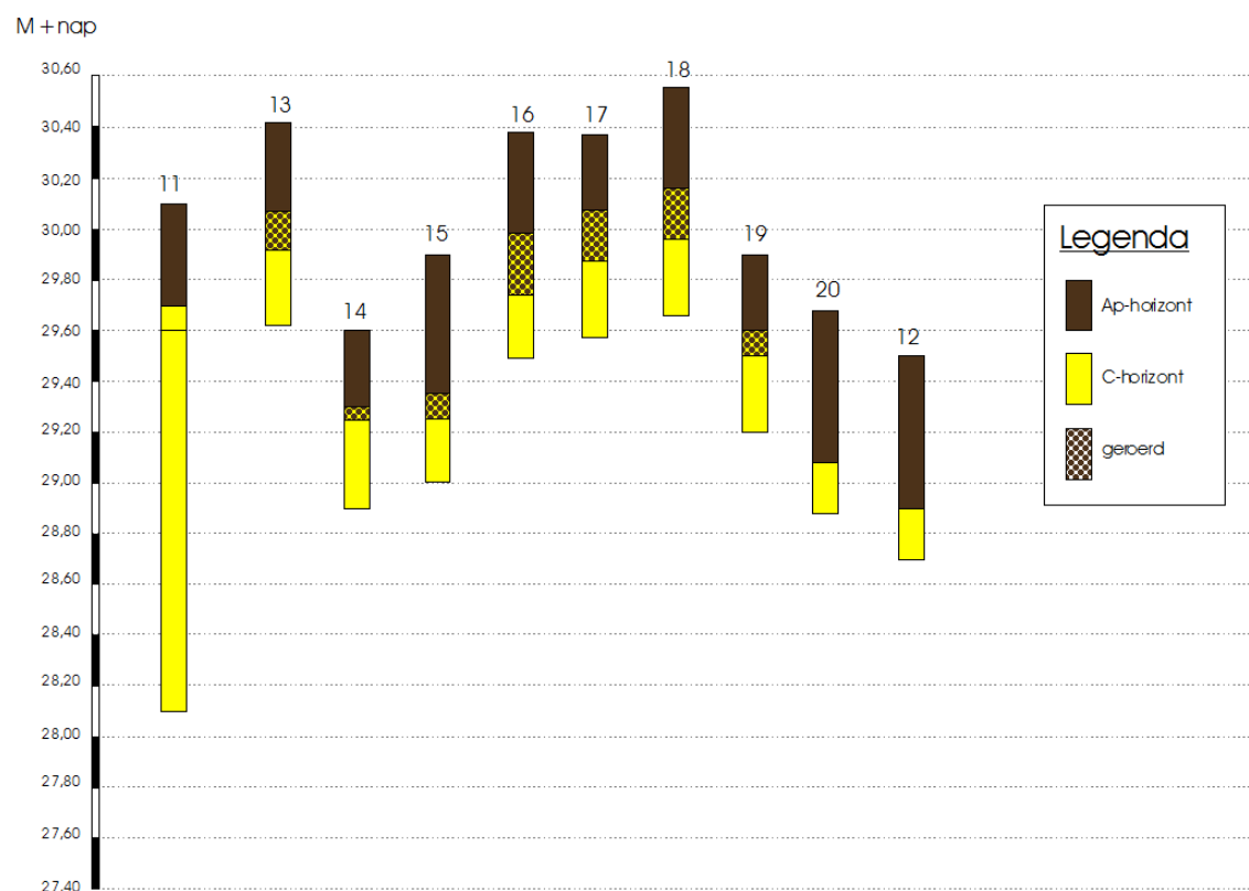
Figuur 18A: Boorprofielen 11-20
