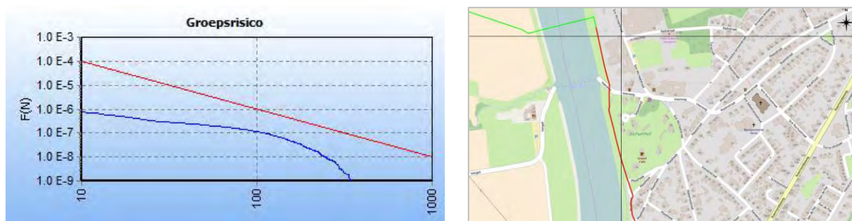
Figuur 9 FN-curve van de kilometer met de hoogste overschrijdingsfactor van gastransportleiding Z-513-20 in de huidige situatie. De ligging van deze kilometer is hiernaast in het rood weergegeven op een topografische kaart.
