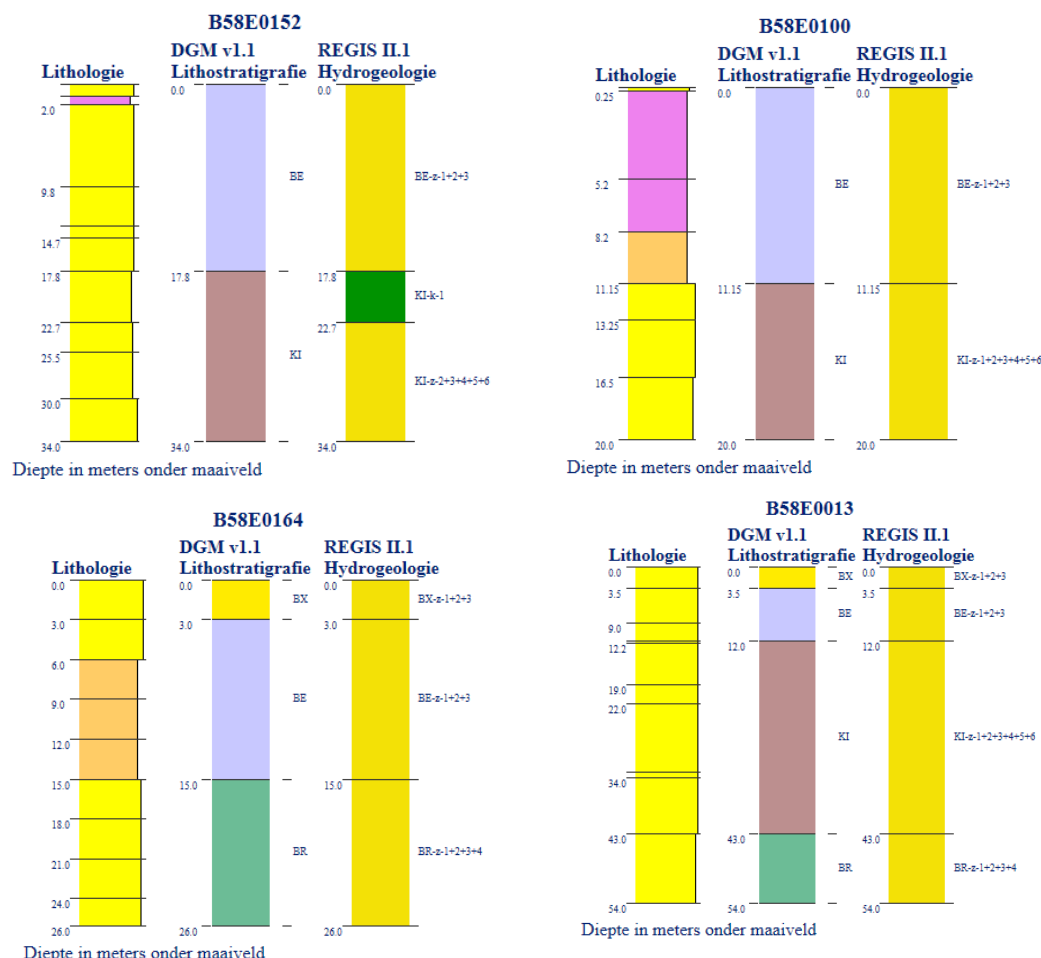
Figuur 4.5: bodempopbouw
