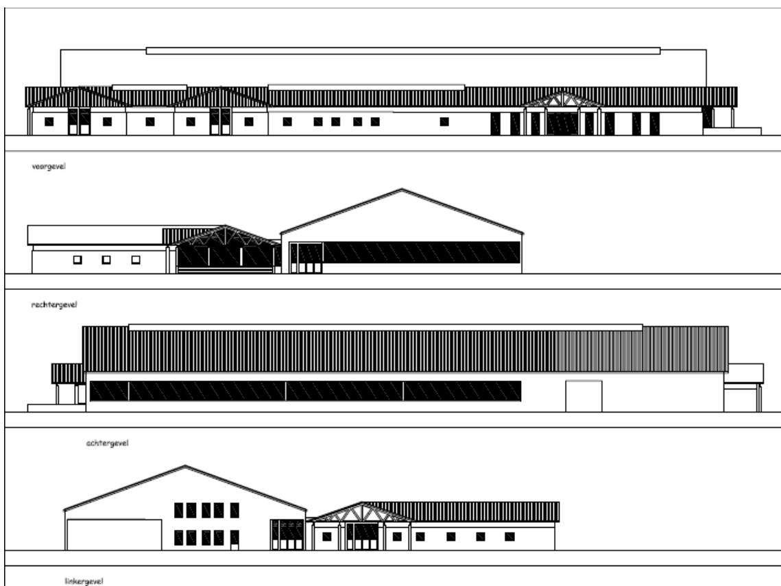
Figuur 7 schetsen gevelaanzichten nieuwbouw Keizersbaan 7a
