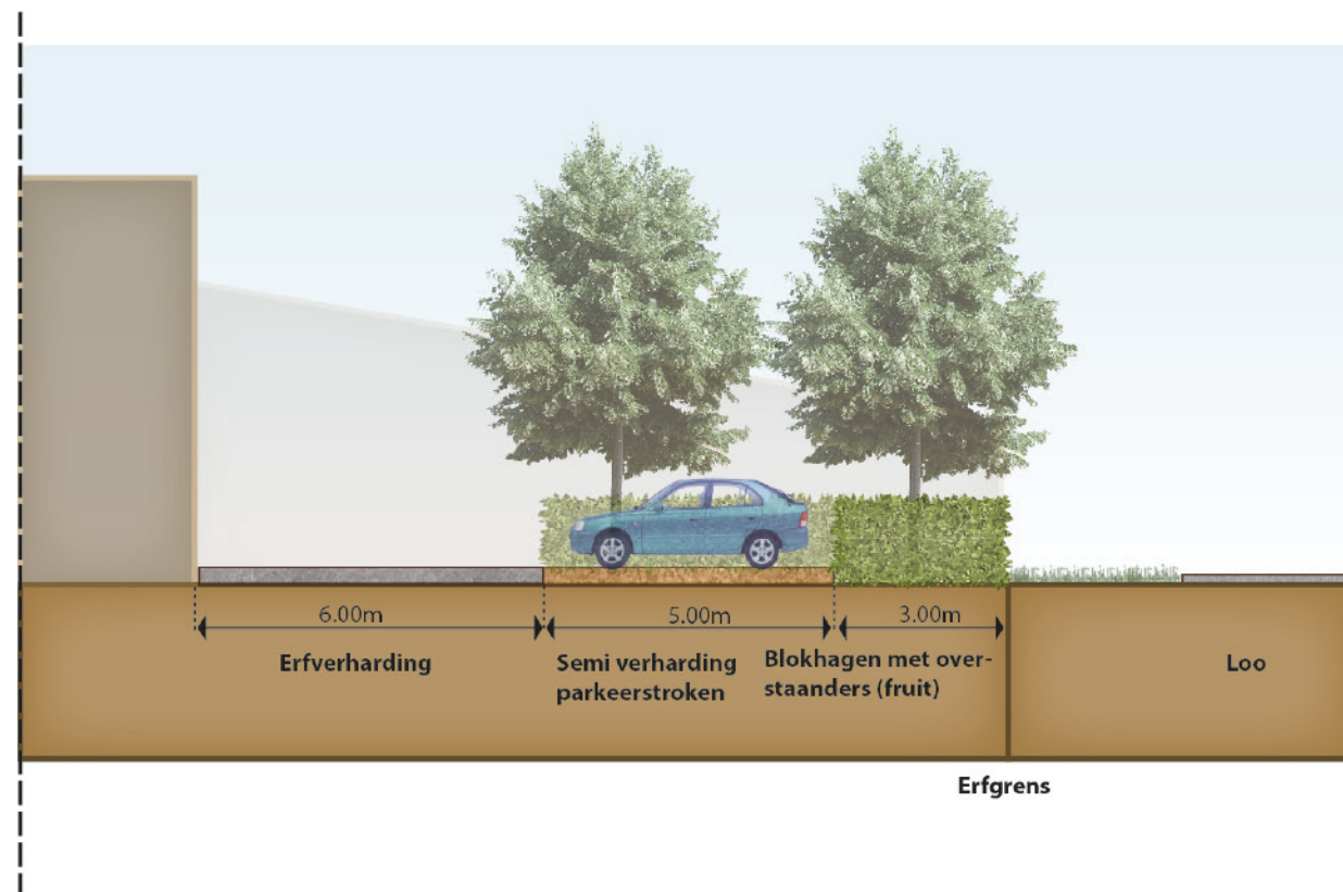
Doorsnede B-B' Doorsnede zijde Loo - 18 juli 2017
