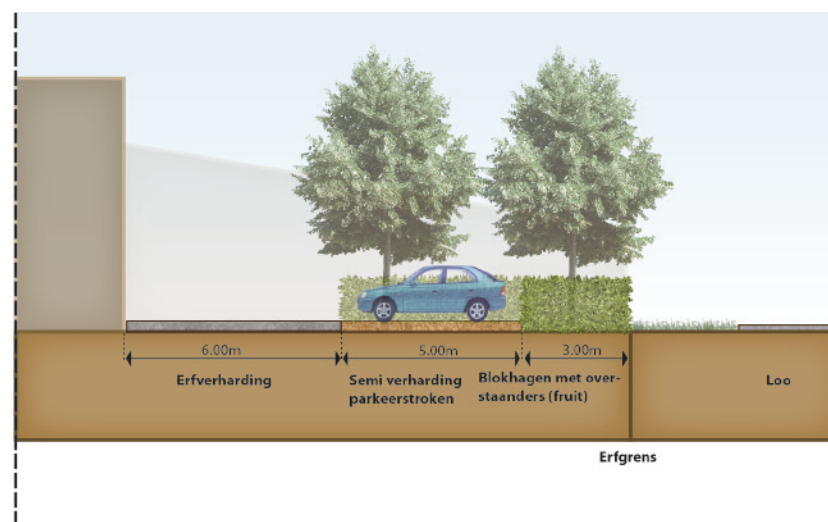
Doorsnede B-B' Doorsnede zijde Loo - 18 juli 2017
