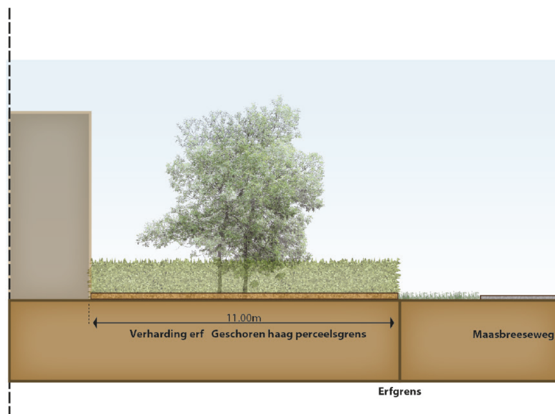
Doorsnede C-C' Doorsnede zijde Maasbreeseweg - 18 juli 2017
