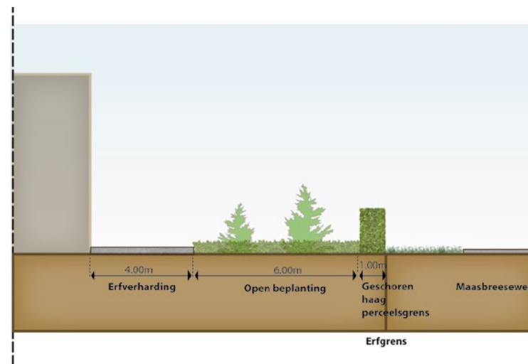
Doorsnede C-C' Doorsnede zijde Maasbreeseweg - 30 januari 2023
