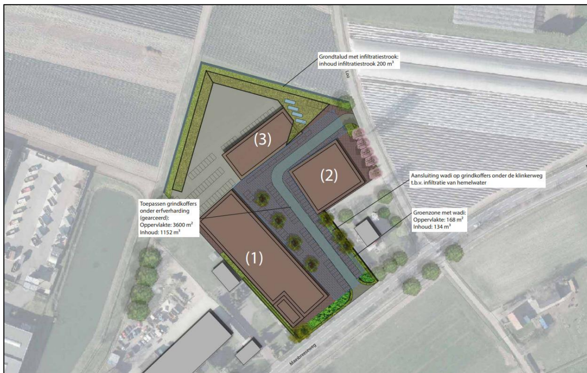
Uitsnede infiltratievoorzieningen
