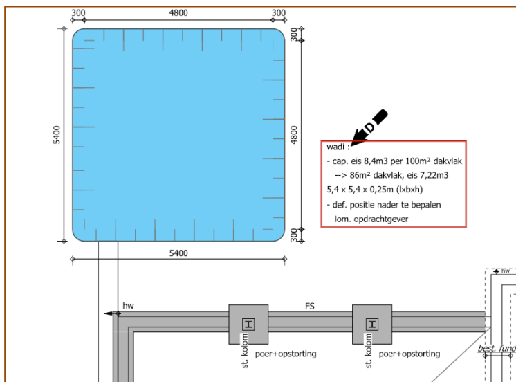
Afbeelding 7: opvang/infiltratie hemelwater
