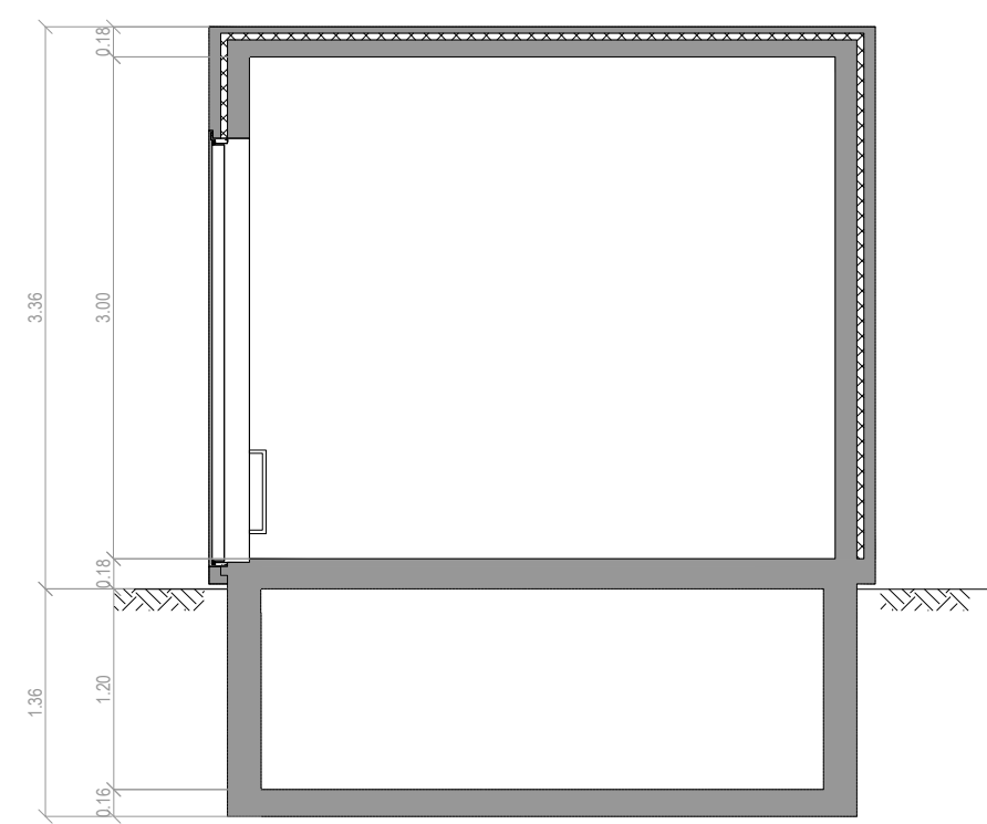
Doorsnede A-A/Cross section A-A
