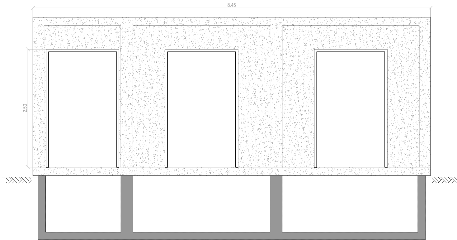
Doorsnede A-A/Cross section A-A
