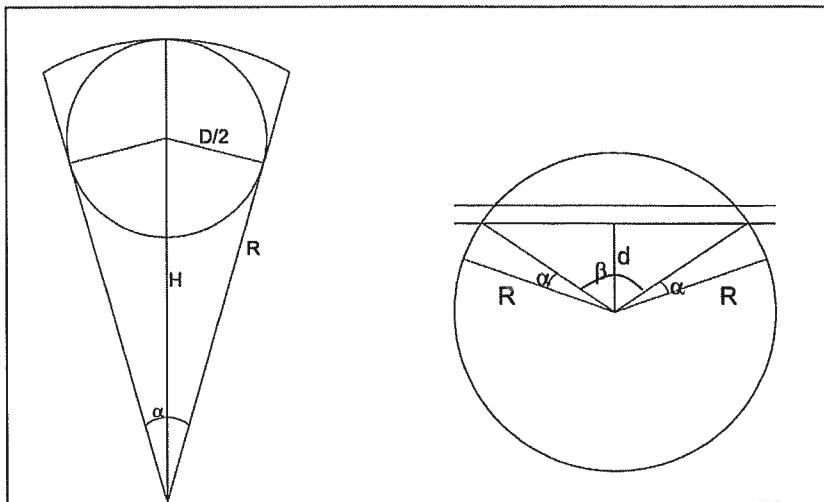
Figuur B2.1. Cirkelsegment en trefhoek
