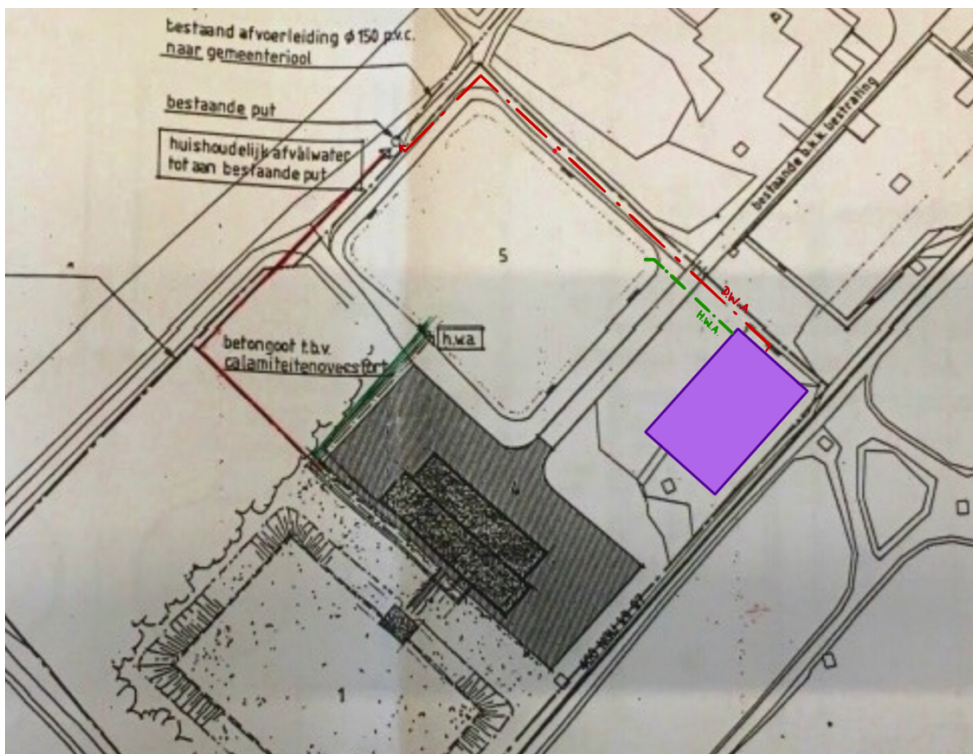
Figuur 8 Bestaande riolering en aansluitingsprincipe HWA en DWA nieuwbouwoods
