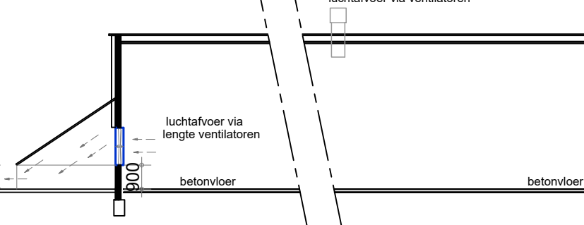
- Langsdoorsnede gebouw 6 -
