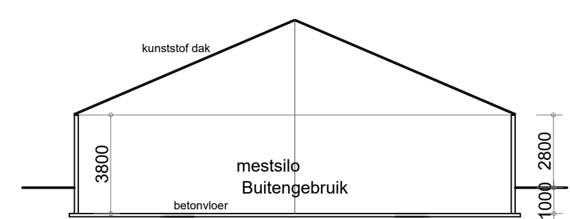
- Doorsnede G - G gebouw 7 -
