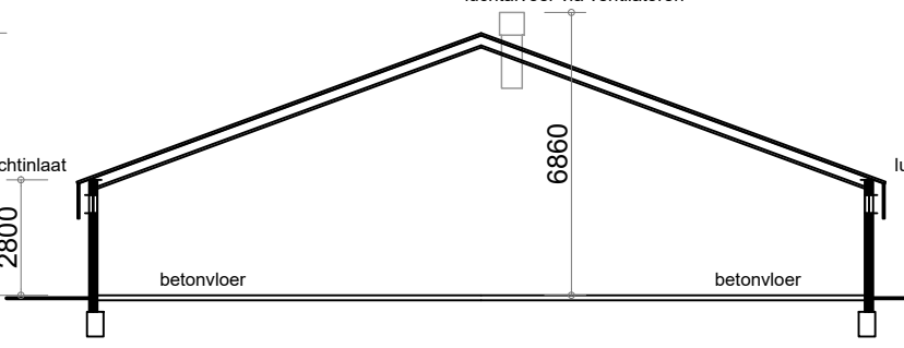
- Doorsnede F - F gebouw 6 -
