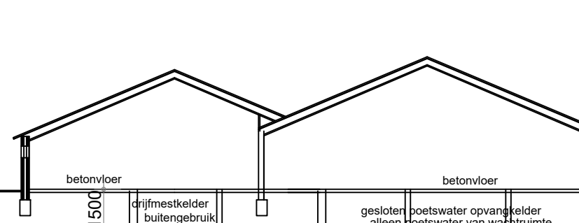
- Doorsnede C - C gebouw 3 -
