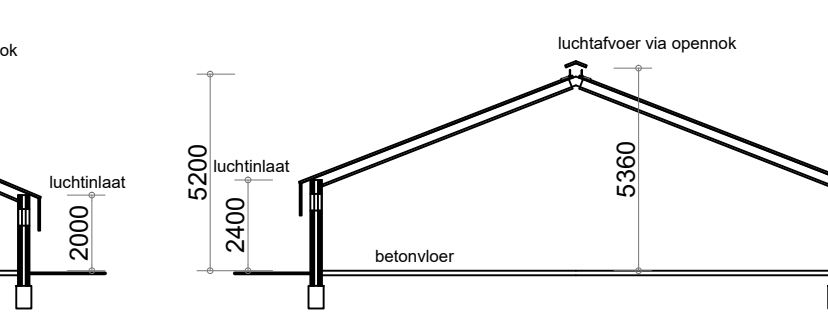
- Doorsnede E - E gebouw 5 -
