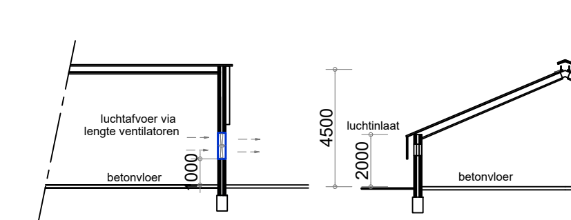
- Langsdoorsnede geb 4 -
