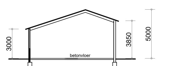
- Doorsnede H - H gebouw 8 -
