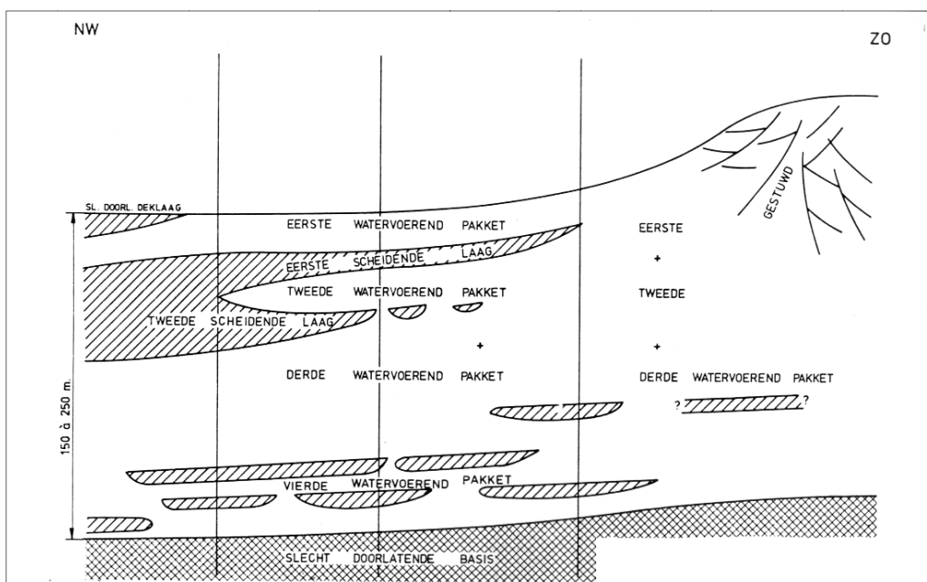
Afbeelding 9. Geohydrologische doorsnede noordwest-zuidoost (bron: Landinrichtingsdienst, 1989)
