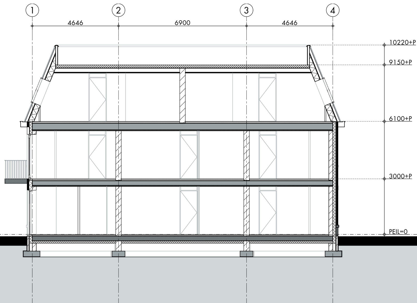
DOORSNEDE A-A
