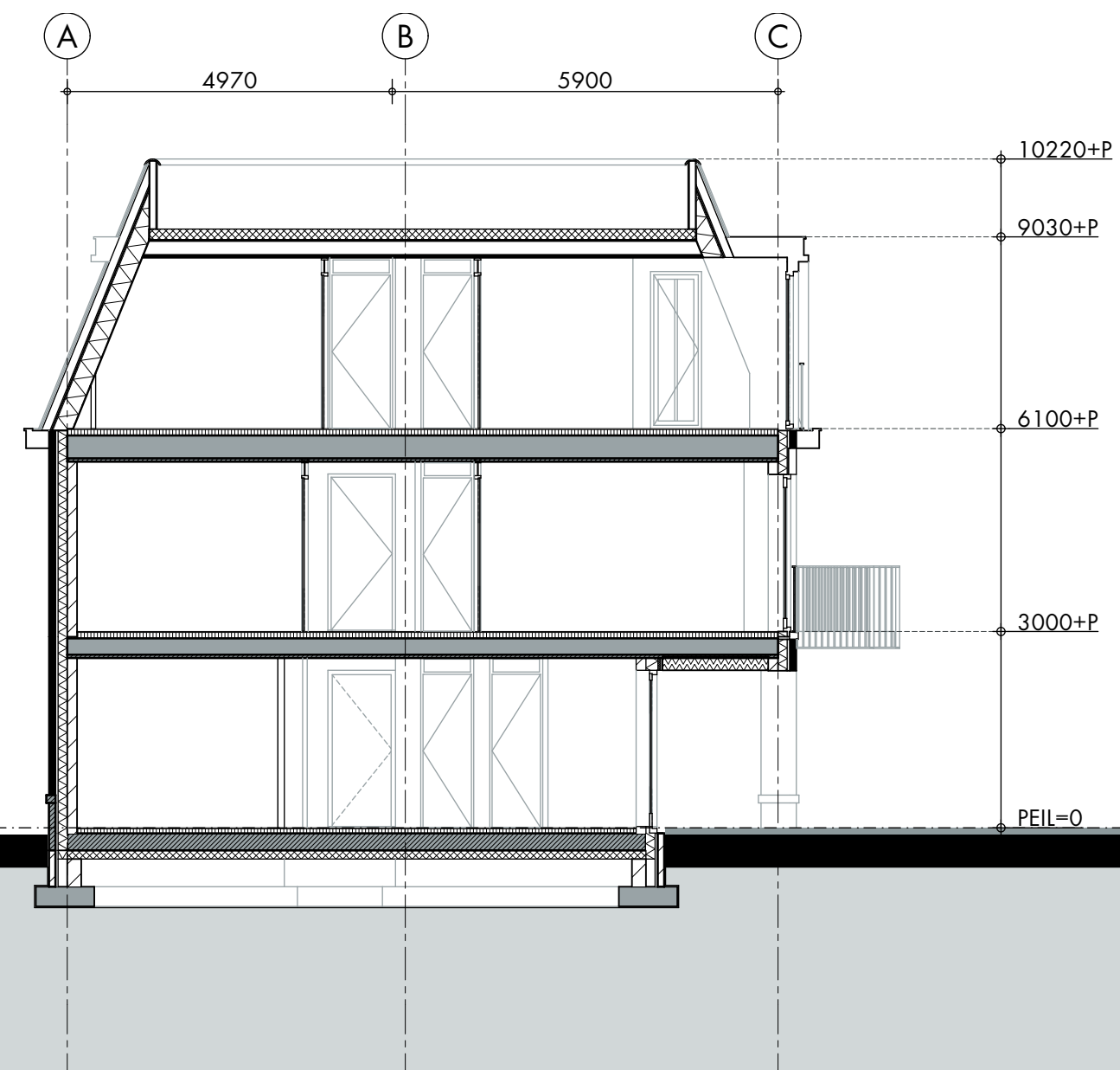
DOORSNEDE B-B
