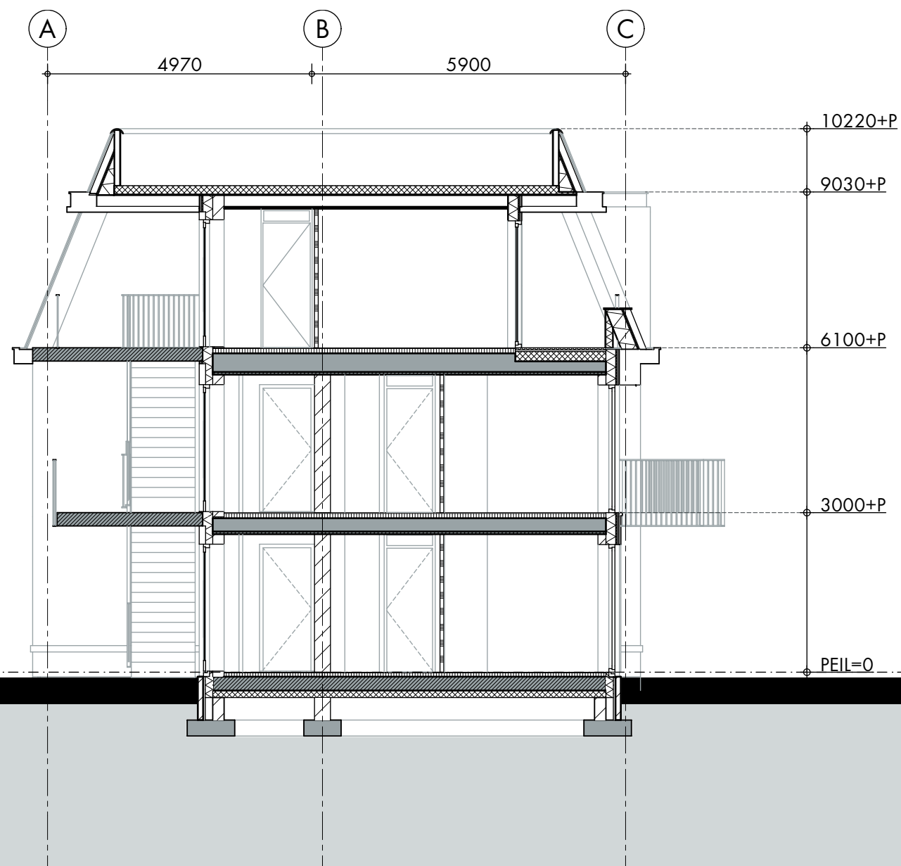
DOORSNEDE C-C
