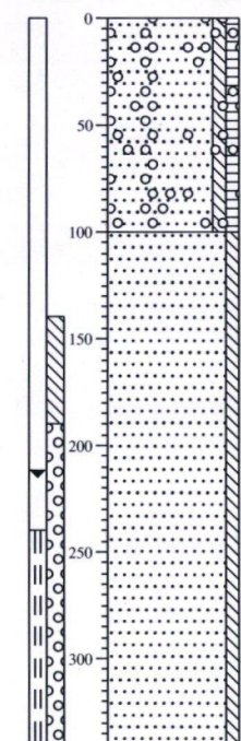
Boring: 12 Datum: 05-05-2014
