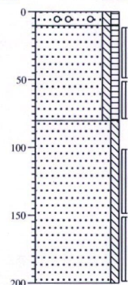
Boring: 7 Datum: 05-05-2014
