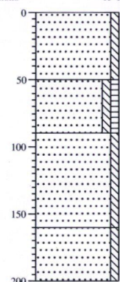
Boring: 10 Datum: 05-05-2014
