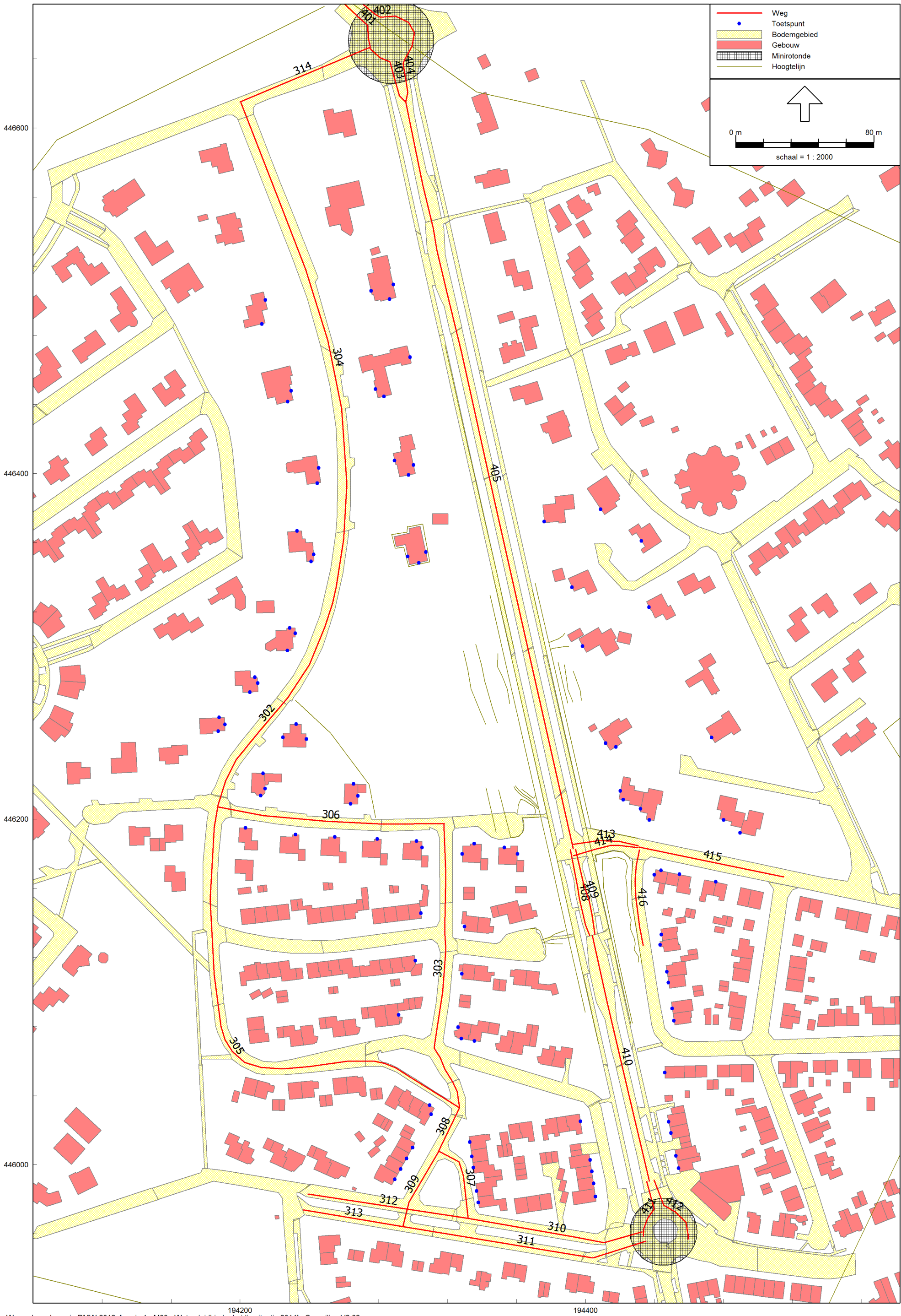
Figuur 4 Overzicht rekenmodel Wet geluidhinder huidige situatie 2014 met ligging wegen
