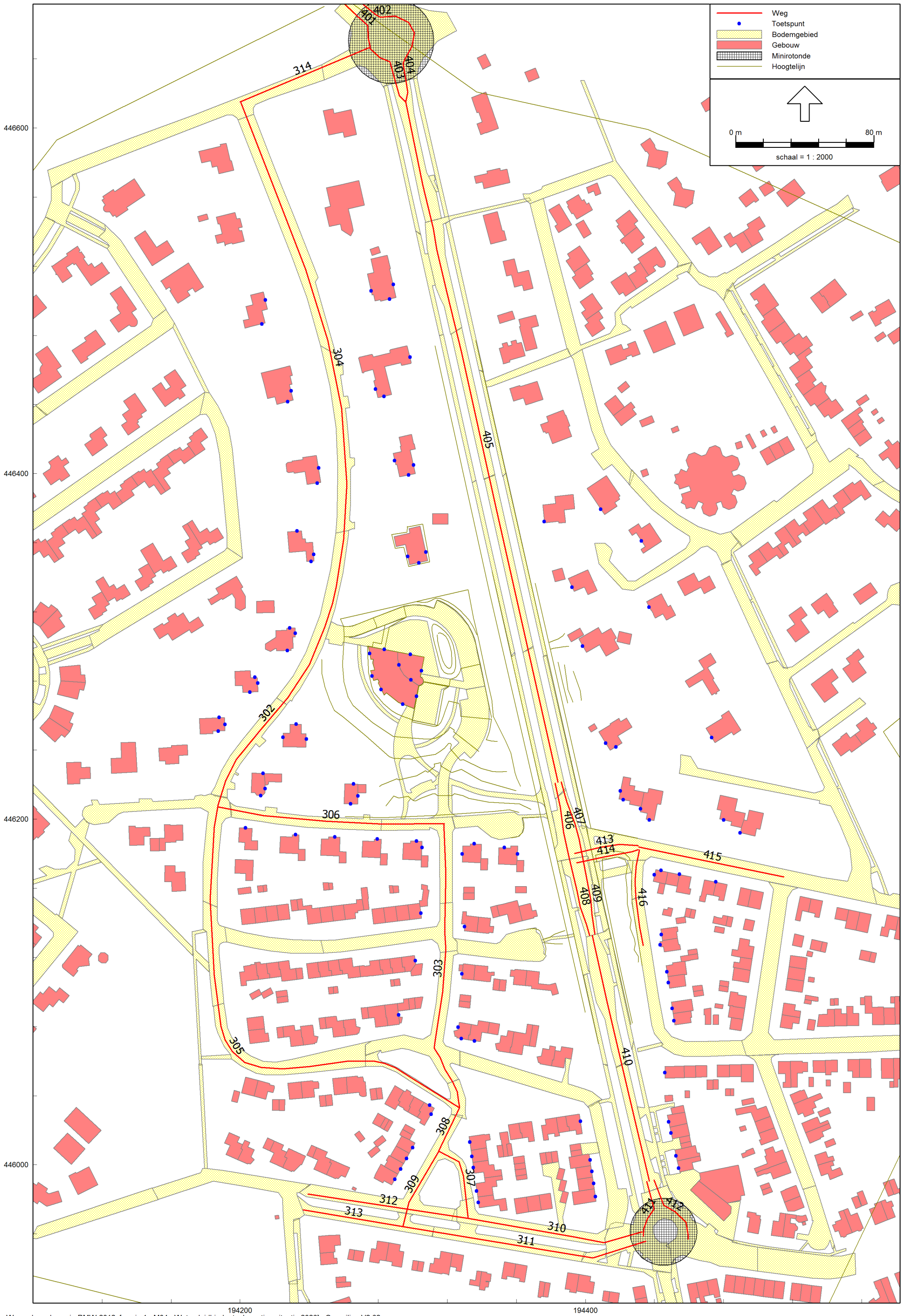
Figuur 5 Overzicht rekenmodel Wet geluidhinder toekomstige situatie 2026 met ligging wegen
