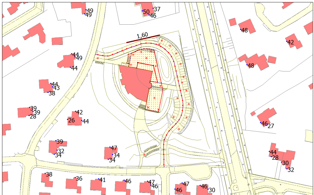
Figuur 5 Schermmaatregel om te voldoen aan de grenswaarde van 50 dB(A)
