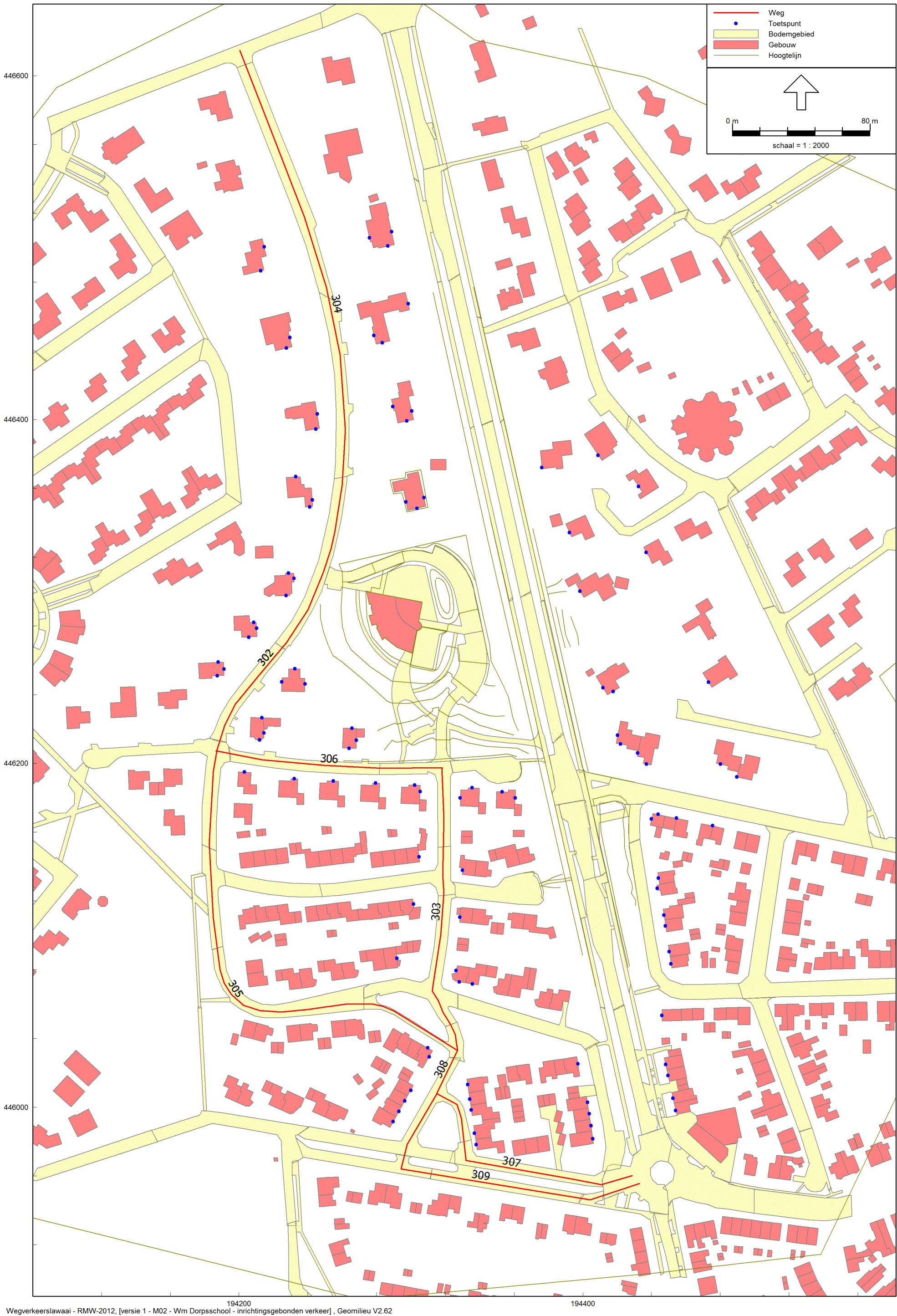
Figuur 3 Overzicht rekenmodel Wet milieubeheer inrichtingsgebonden verkeer Dorpschool met ligging wegen
