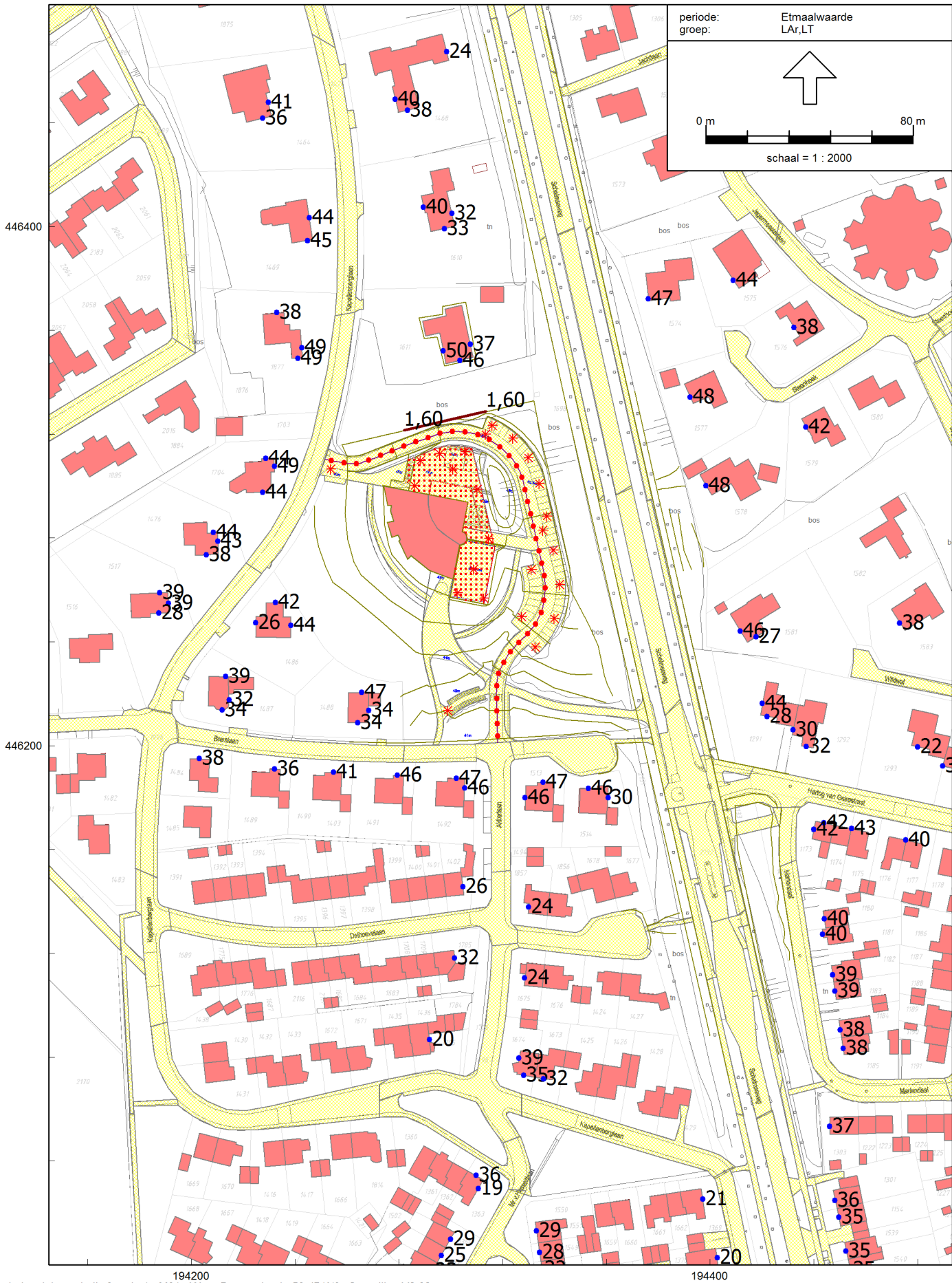
Figuur 7 Langtijdgemiddelde beoordelingsniveau LAR,LT t.g.v. Dorpschool Maatregelen 50 dB(A)
