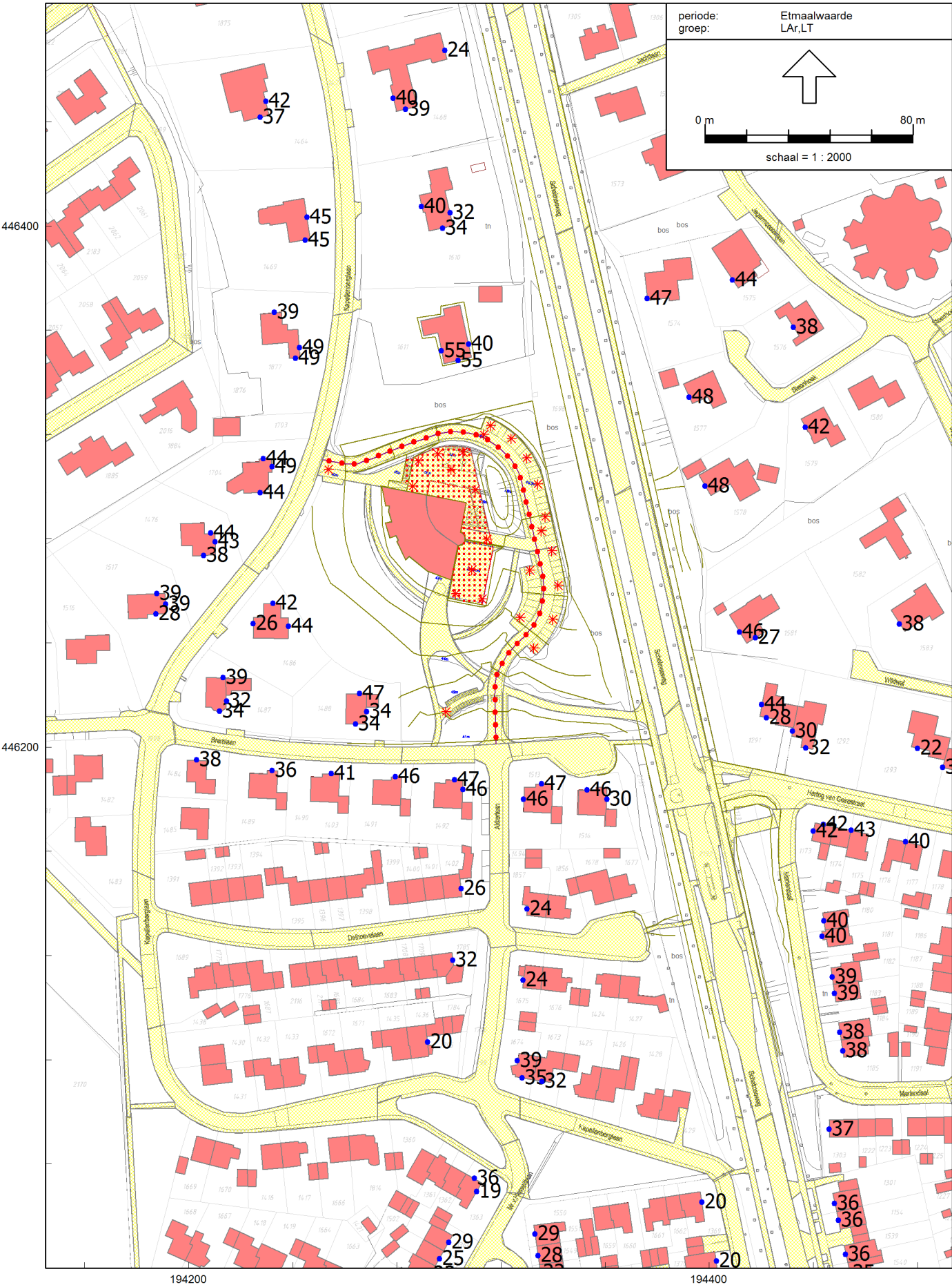
Figuur 6 Langtijdgemiddelde beoordelingsniveau LAR,LT t.g.v. Dorpschool Zonder maatregelen
