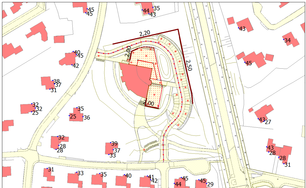
Figuur 6 Schermmaatregel om te voldoen aan de richtwaarde van 45 dB(A)
