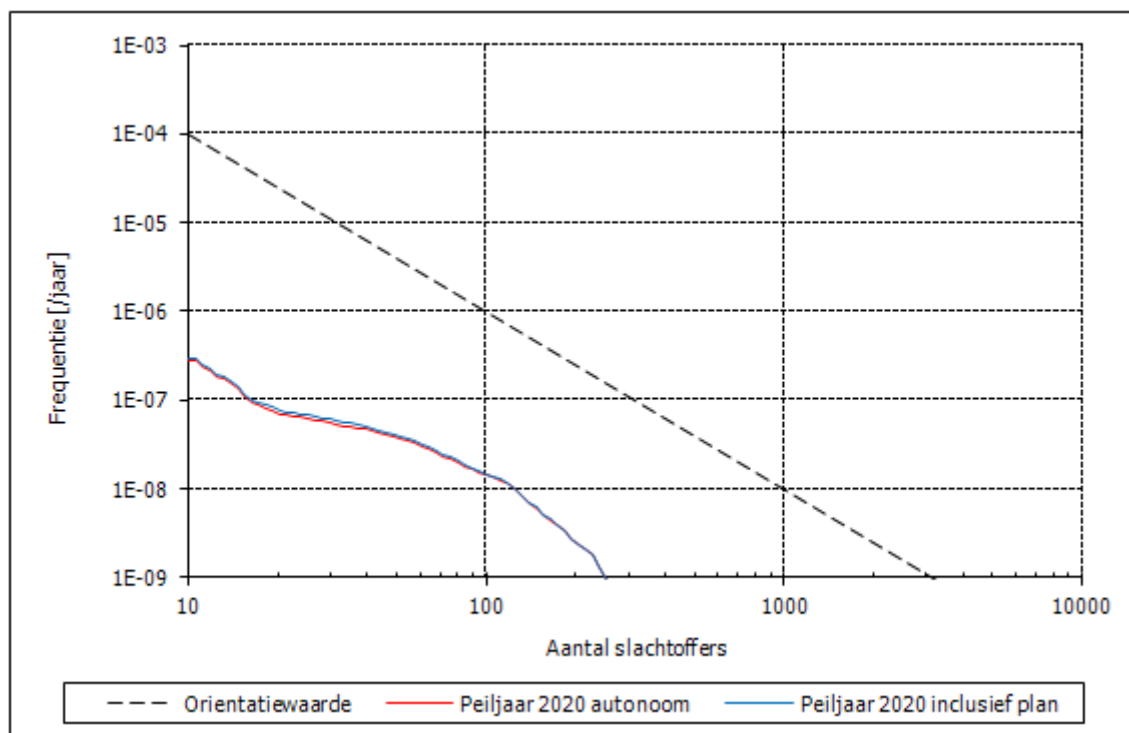
Figuur 6. Groepsrisicografiek A12 in de autonome ontwikkeling (rood) en de situatie met planontwikkeling (blauw) in de toekomstige situatie (Global Economy scenario).
