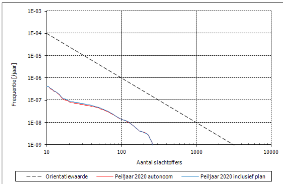
Figuur 5. Groepsrisicografiek A12 in de autonome ontwikkeling (rood) en de situatie met planontwikkeling (blauw) bij maximale benutting van de groeiruwte van het transport.
