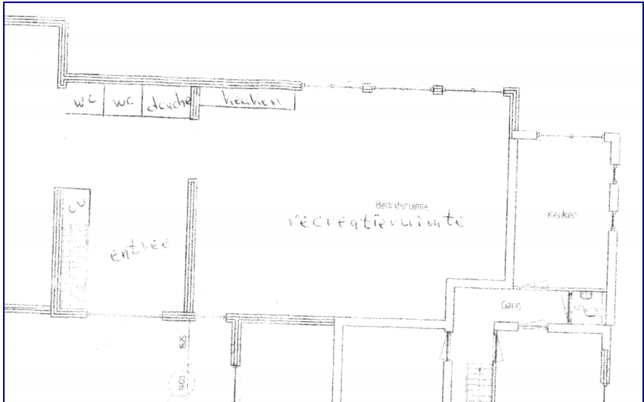
Afbeelding 3. Plattegrond cursusruimte (begane grond)
