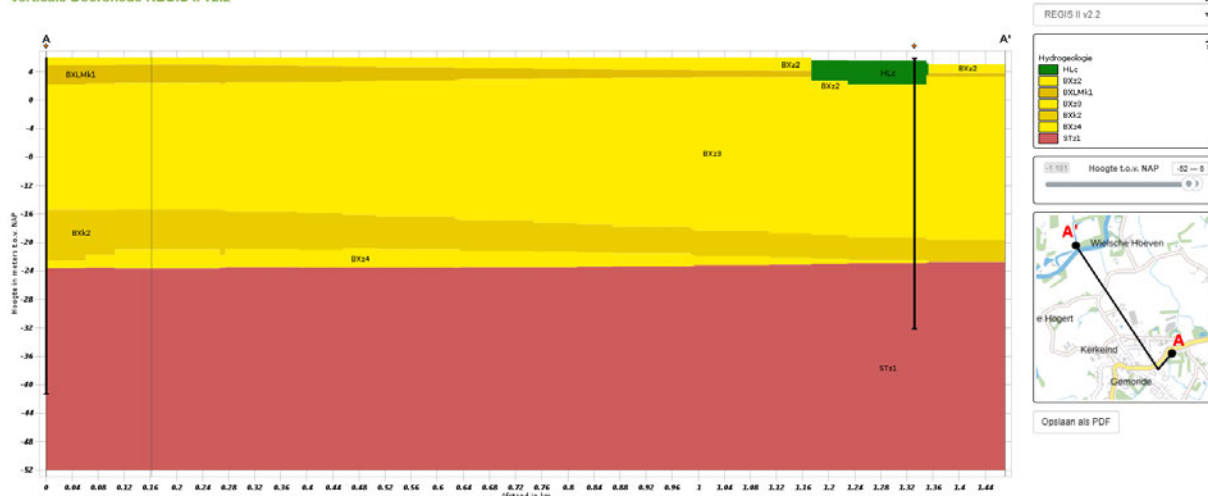
Verticale Doorsnede REGIS II v2.2
