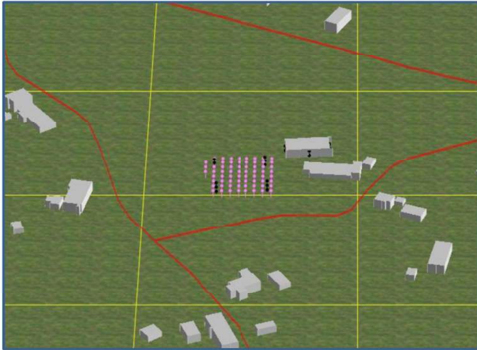
Afbeelding 4. Rekenmodel, 3d-weergave
