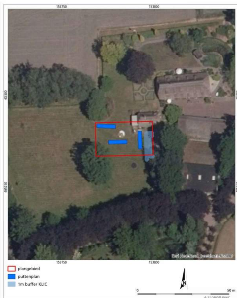
Afb. 2.1 Puttenplan
