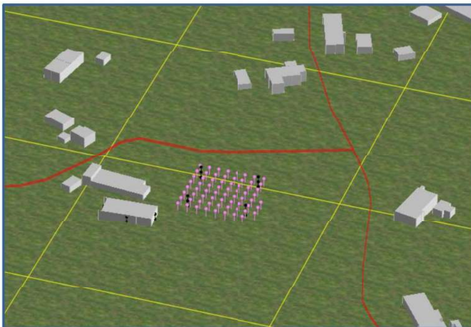
Afbeelding 5. Rekenmodel, 3d-weergave
