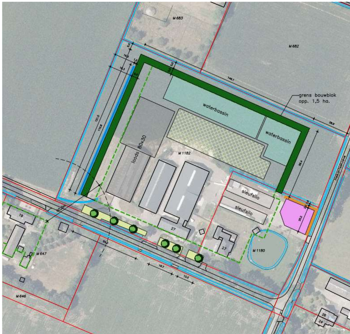
Situatietekening gewenste situatie. Bron: DLV Advies.
