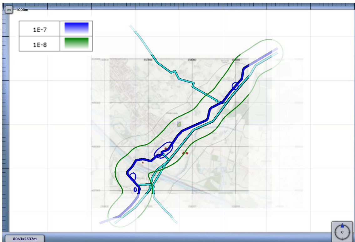
3.3 Figuur 3.3 Plaatsgebonden risico voor 8202_leiding-A-527-deel-1 van N.V. Nederlandse Gasunie
