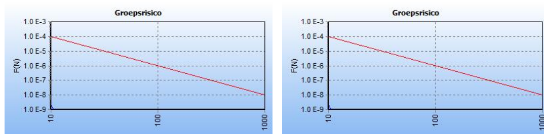
Figuur 3. Groepsrisico A-525, huidig (links) en toekomstig (rechts)
