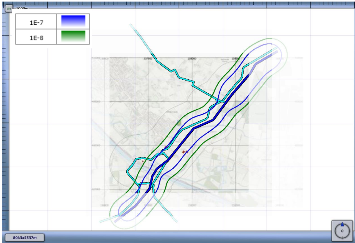
3.2 Figuur 3.2 Plaatsgebonden risico voor 8202_leiding-A-526-deel-1 van N.V. Nederlandse Gasunie
