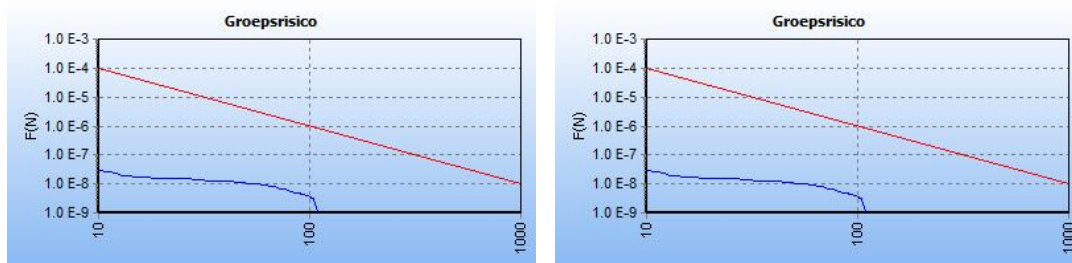
Figuur 5. Groepsrisico A-527, huidig (links) en toekomstig (rechts)
