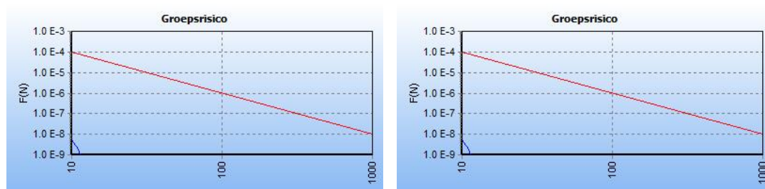
Figuur 4. Groepsrisico A-526, huidig (links) en toekomstig (rechts)
