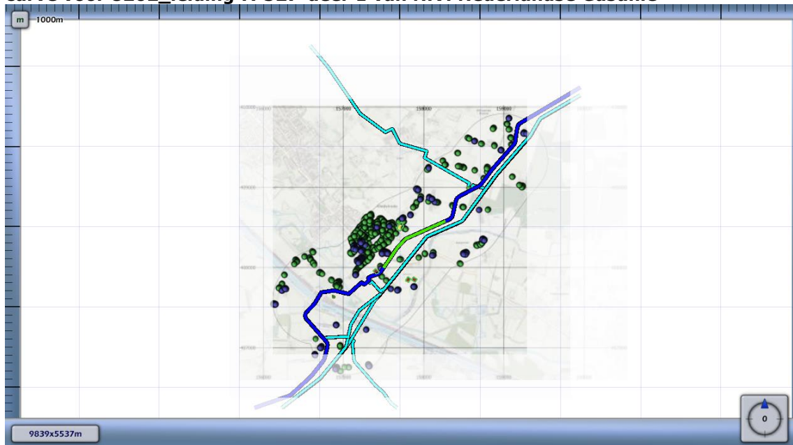
Figuur 4.6 Kilometer leiding behorende bij de maximale overschrijding van de FN-curve voor 8202_leiding-A-527-deel-1 van N.V. Nederlandse Gasunie
