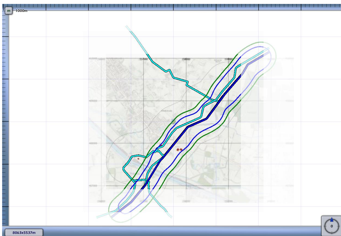
3.1 Figuur 3.1 Plaatsgebonden risico voor 8202_leiding-A-525-deel-1 van N.V. Nederlandse Gasunie
