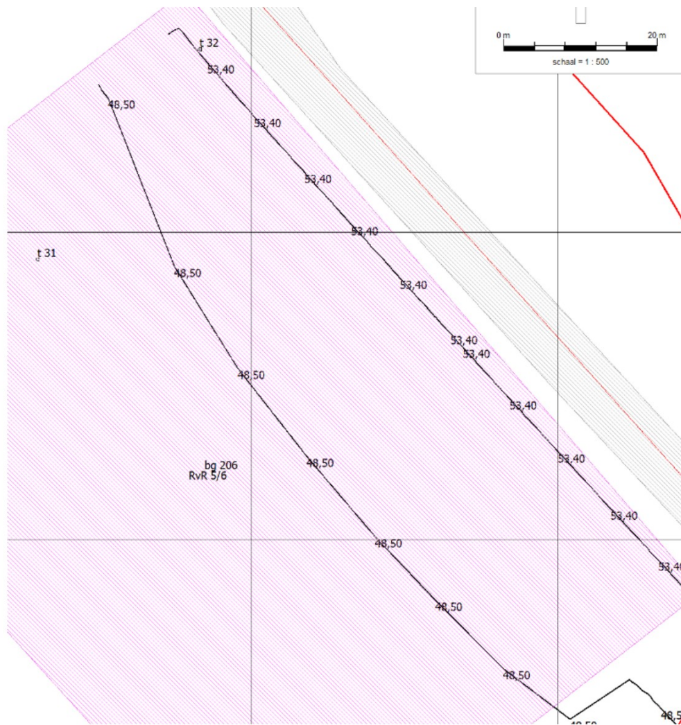
Geluidbelastingen Lden (incl. aftrek art 110g Wgh) Nieuweweg. Ligging van de 53 en 48 dB contour..
