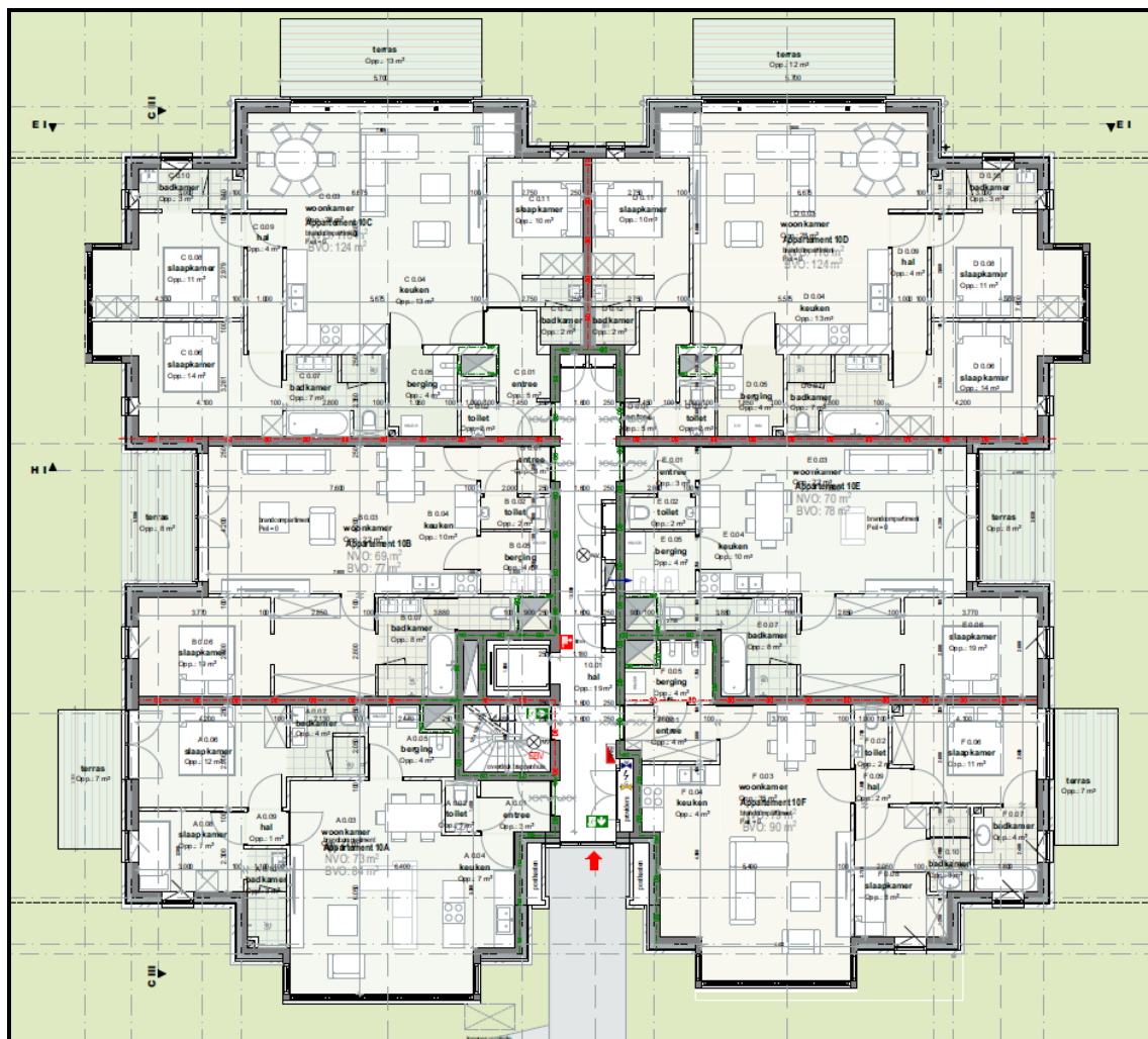
Figuur 6: Indeling begane grond Hampton 1
