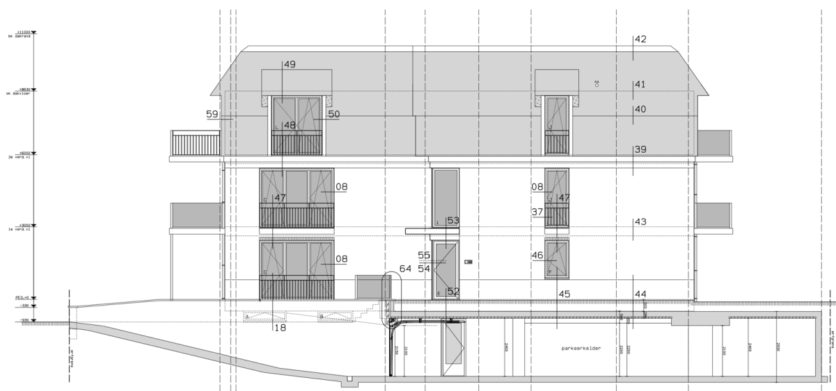
Figuur 13: Aanzicht gebouw 2 westzijde beoogde situatie (bron: VO Vlamingpolderweg 2, Mark Architecten)
