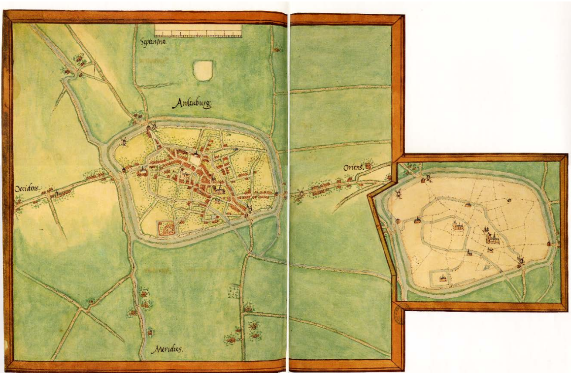
Afbeelding 2 Stad Aardenburg getekend door Jacob van Deventer. Hierop zijn de middeleeuwse vestingwerken goed zichtbaar (Bron: Jacob van Deventer, 1565)
