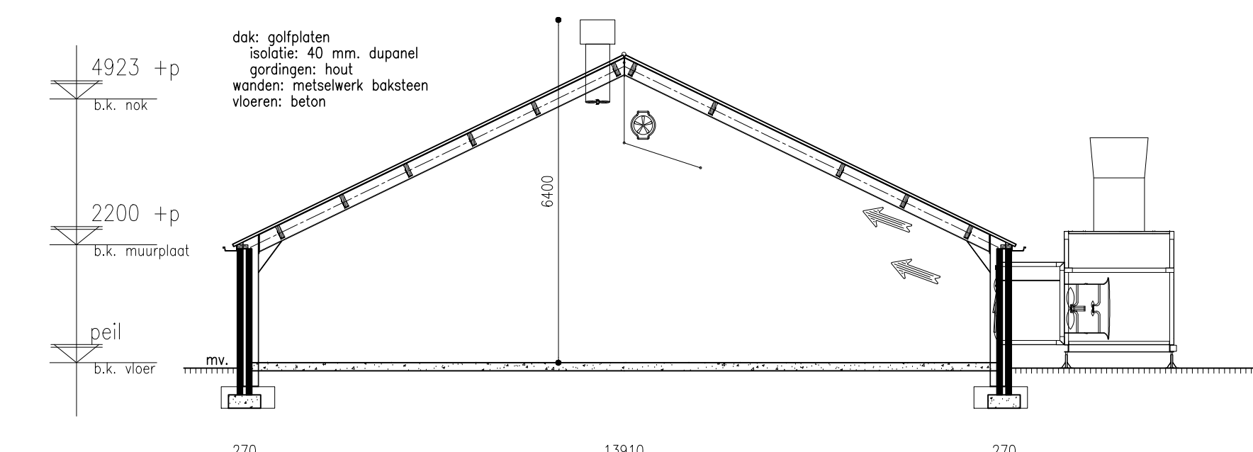
doorsnede A-A
