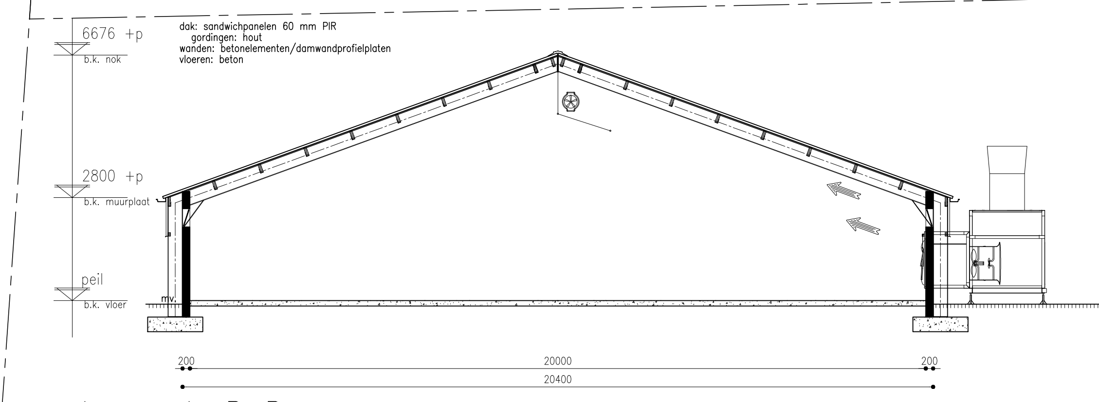
doorsnede B-B
