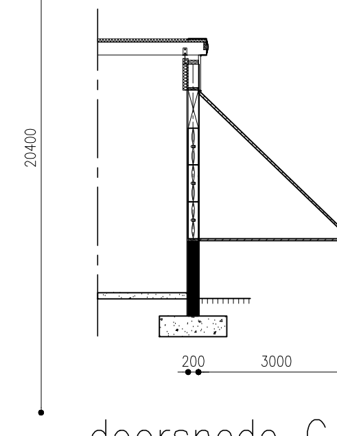
doorsnede C-C
