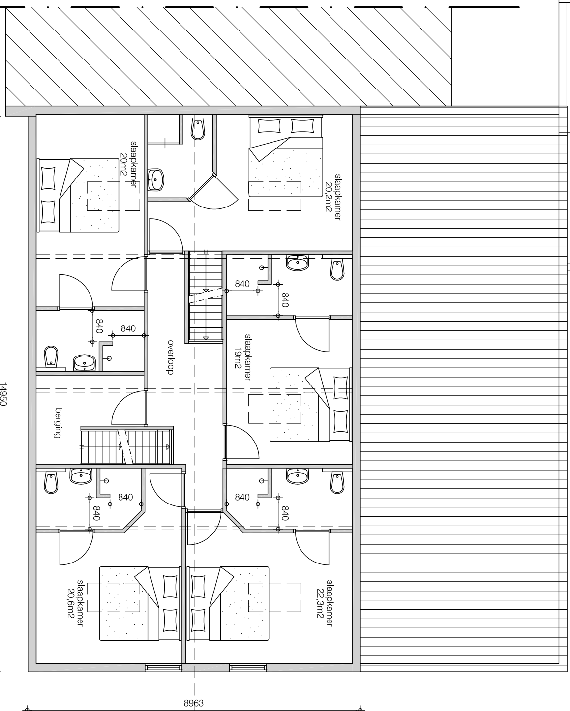
VERDIEPING NIEUW
