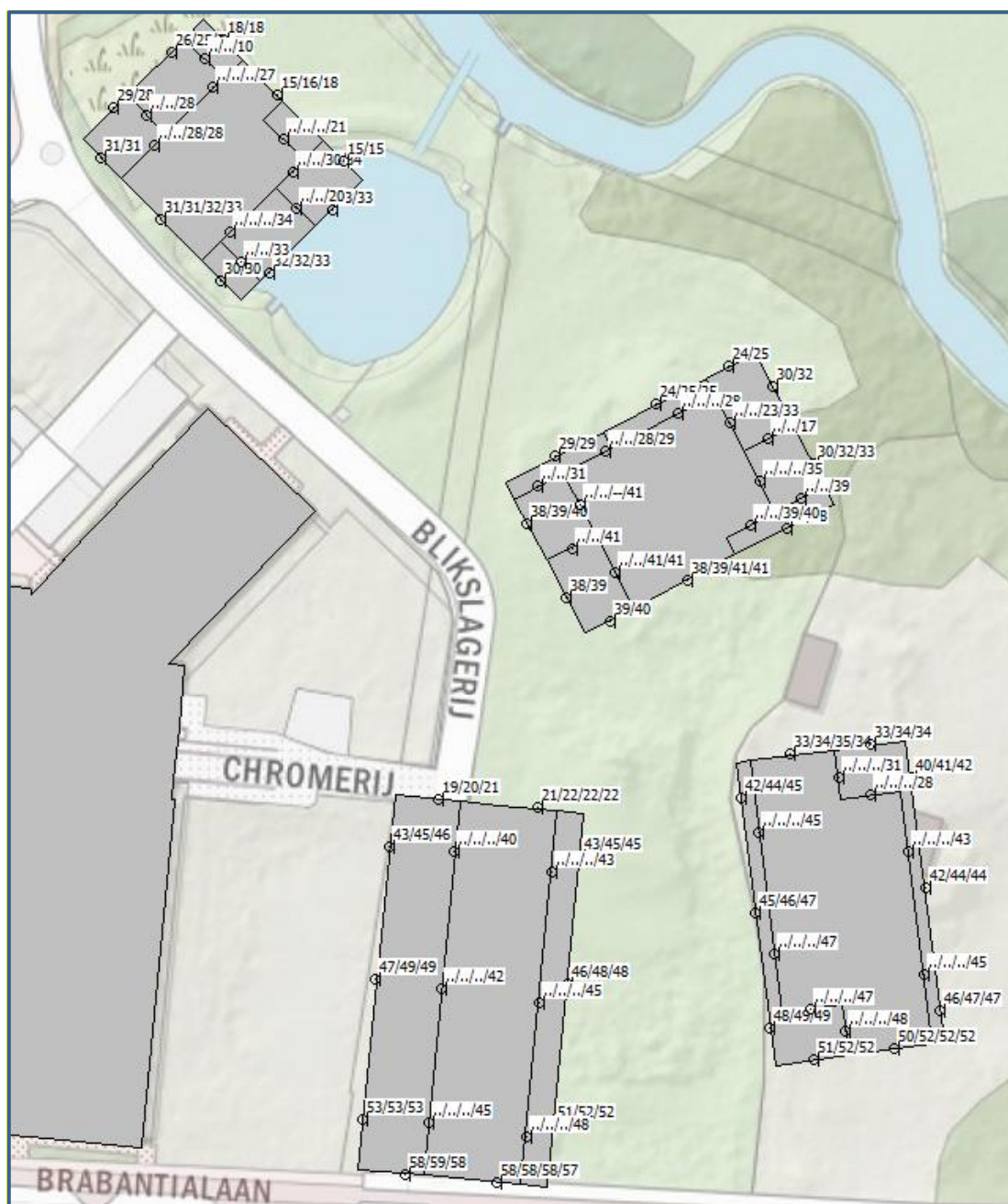
Afbeelding 8. Geluidbelastingen Lden (incl. aftrek art. 110g Wgh) Brabantialaan Berekende geluidbelastingen op een hoogte van 1,5 / 4,5 / 7,5 / 10,5 meter
