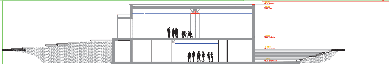
Doorsnede B-B
