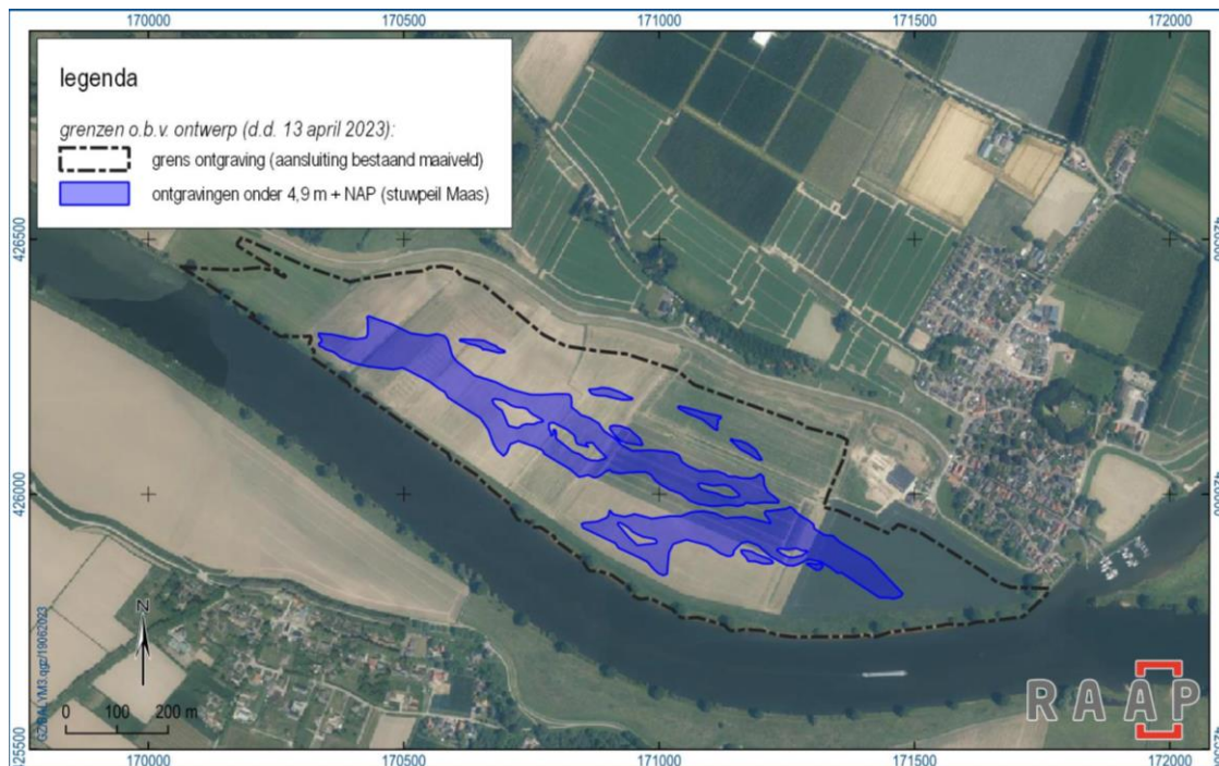
Figuur 3. Ontgravingen onder het stuwpeil van de Maas (cf. ontwerp variant 7 d.d. 13 april 2023).
