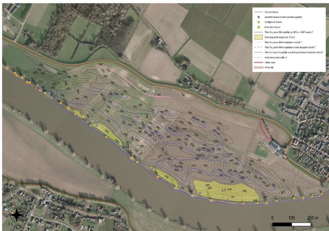
Figuur 1. Ontwerpkaart met hoogtelijnen variant 7 (aanlevering Natuurmonumenten d.d. 13 april 2023).
