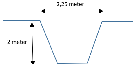
Profiel met waterberging:
