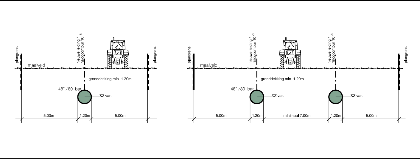
Opbouw leidingstrook schaal 1: 200
