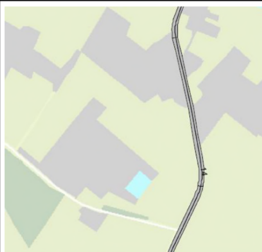
Etmaalintensiteiten
