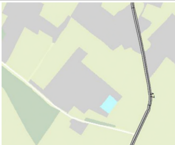
etmaalintensiteiten
