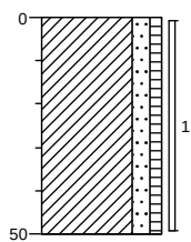
Boring: C03
