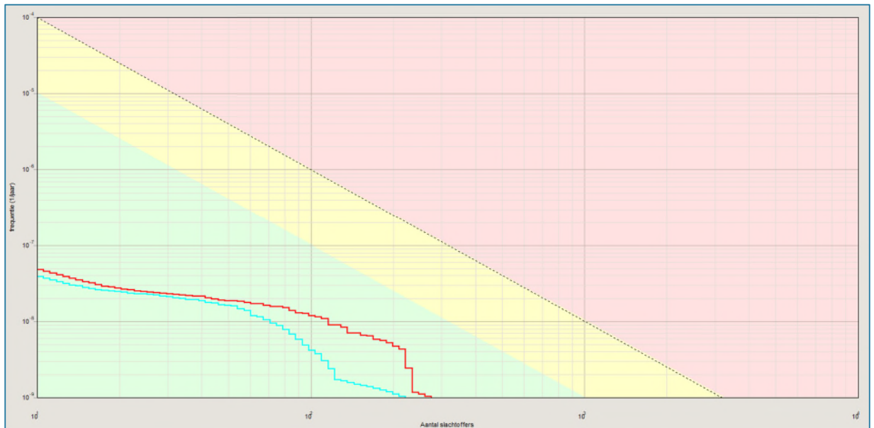
Figuur B2-3 Groepsrisico van de spoorlijn Den Bosch Diezebrug aansl. – Ressen Noord.
