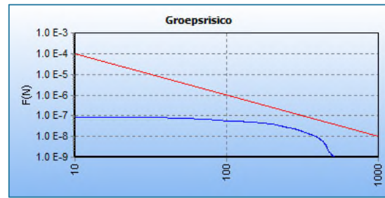
Figuur B1-8 Groepsrisico hogedruk aardgastransportleiding A-533 in de toekomstige situatie
