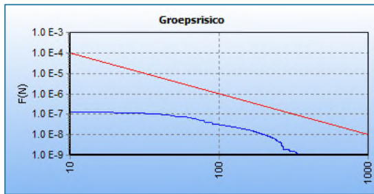
Figuur B1-7 Groepsrisico hogedruk aardgastransportleiding A-533 in de huidige situatie
