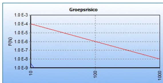
Figuur 3-14 Groepsrisico hogedruk aardgastransportleiding A-674 in de huidige situatie
