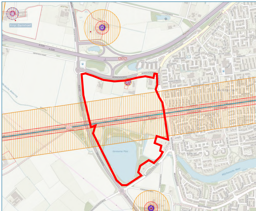
Figuur 3-2 plangebied in relatie tot de propaantank, de Rijksweg A326 en de spoorlijn
