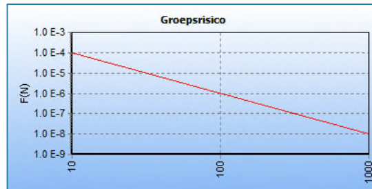
Figuur 3-7 Groepsrisico hogedruk aardgastransportleiding A-507 in de toekomstige situatie
