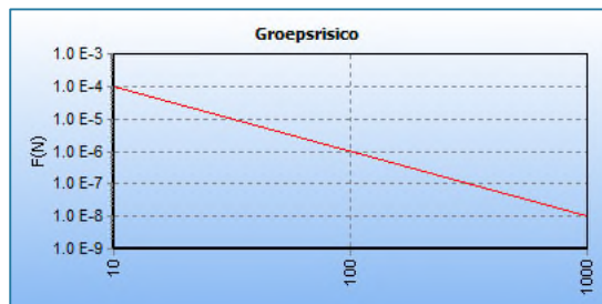
Figuur 3-6 Groepsrisico hogedruk aardgastransportleiding A-507 in de huidige situatie
