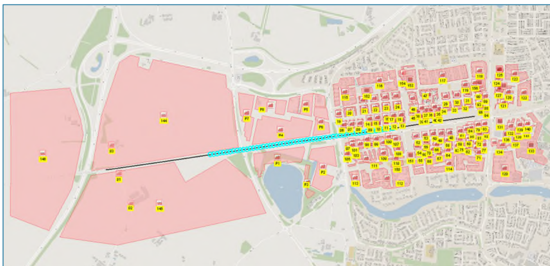
Figuur B2-5 Ligging van de kilometer met het hoogste groepsrisico in de toekomstige situatie (blauw)
