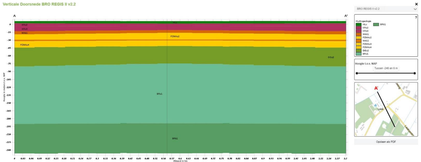
Verticale Doorsnede BRO REGIS II v2.2
