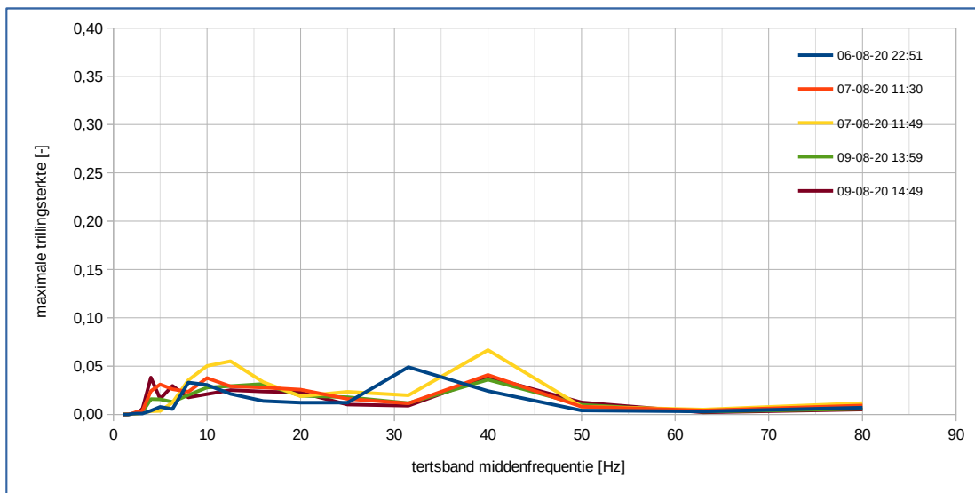
f3.3 Spectrale verdeling van de trillingsterkte als gevolg van de treinpassages (verticale Z richting)
