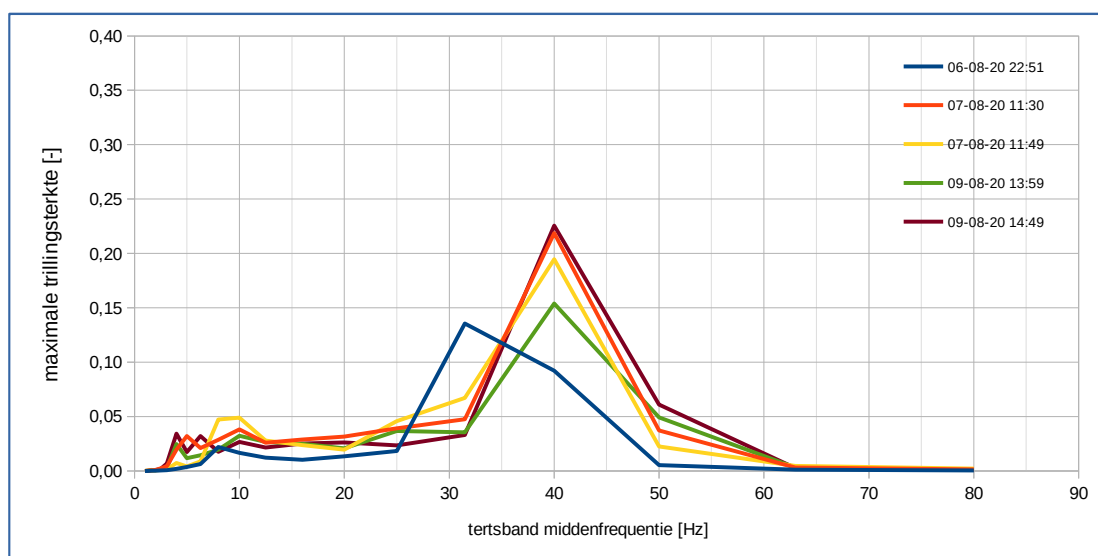
f3.1 Spectrale verdeling van de trillingsterkte als gevolg van de treinpassages (horizontale X richting)
