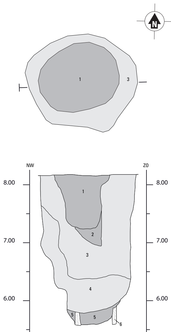
Fig. 17.31. Wijchen-Oostflank. Waterput 7006, Schaal 1:40.
