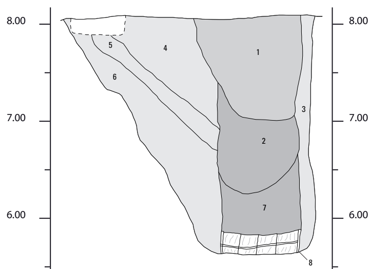
Fig. 17.29. Wijchen-Oostflank. Waterput 7004, Schaal 1:40.
