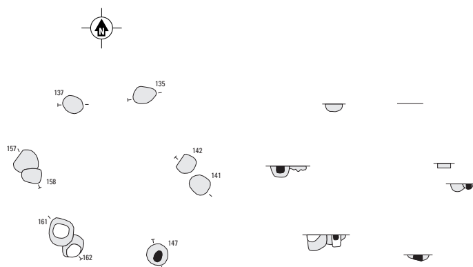
Fig. 17.25. Wijchen-Oostflank. Plattegrond van Roedenberg 13002. Schaal 1:200. NAP 8.50.
