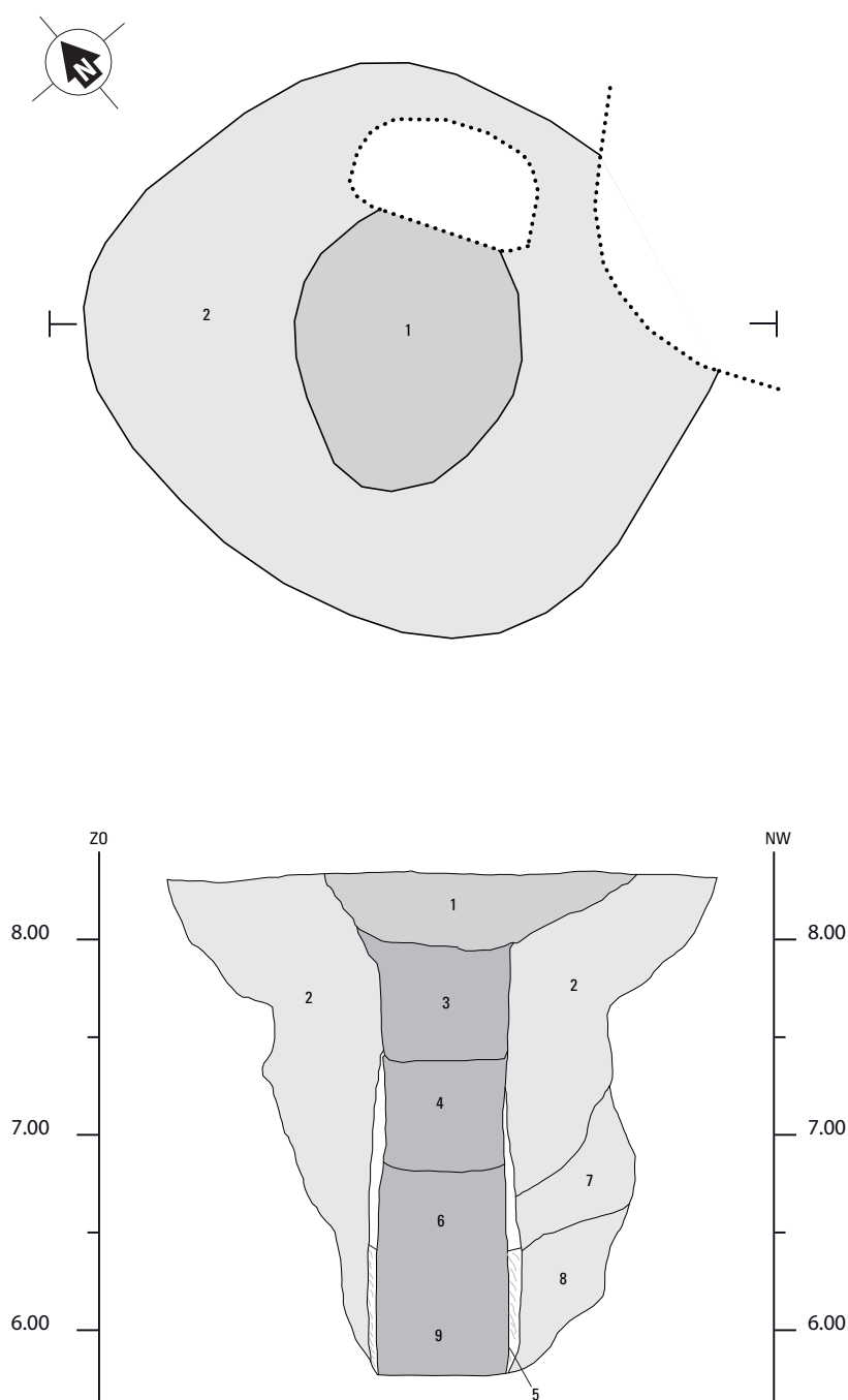
Fig. 17.28. Wijchen-Oostflank. Waterput 7003, Schaal 1:40.
