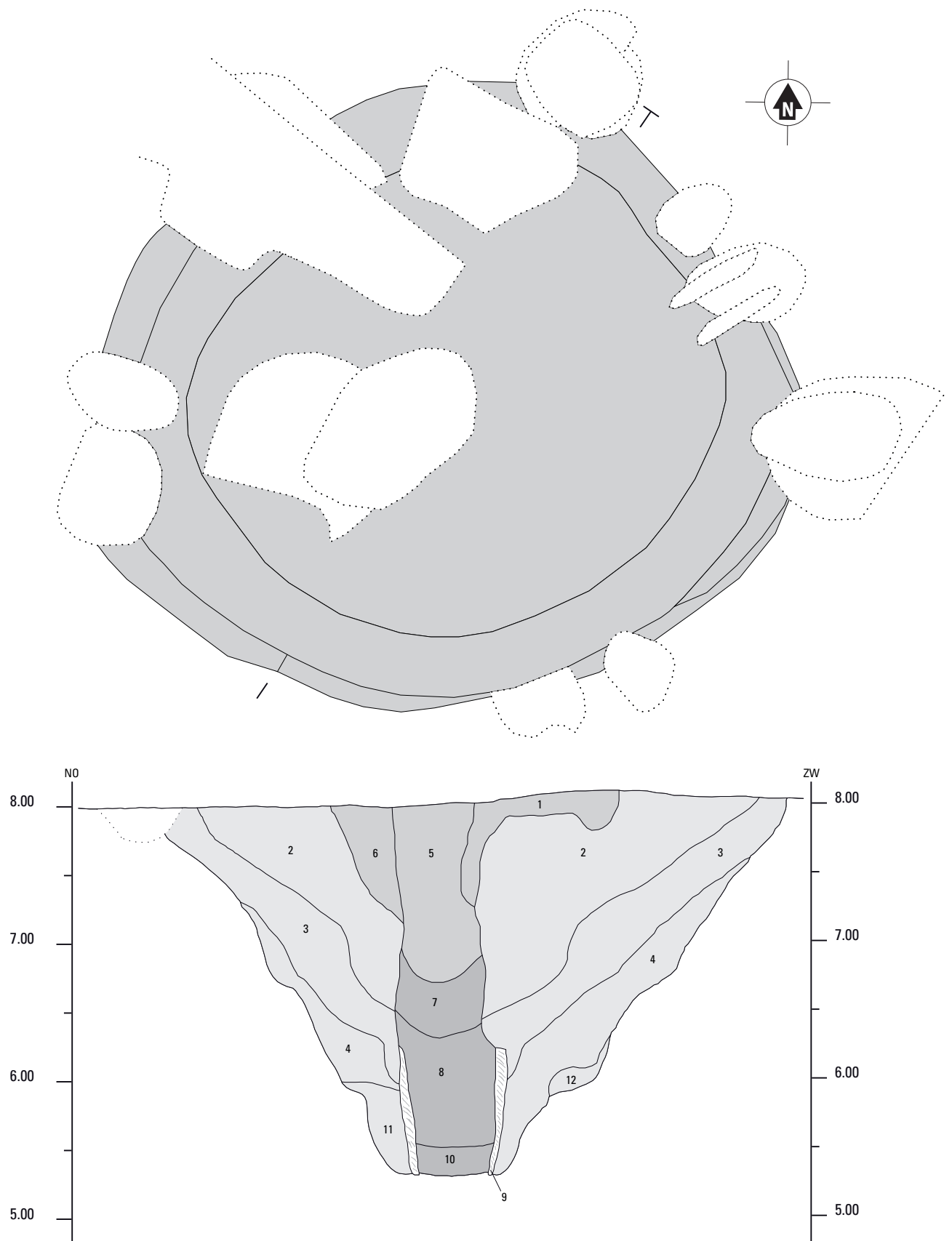
Fig. 17.26. Wijchen-Oostflank. Waterput 7001, Schaal 1:40.
