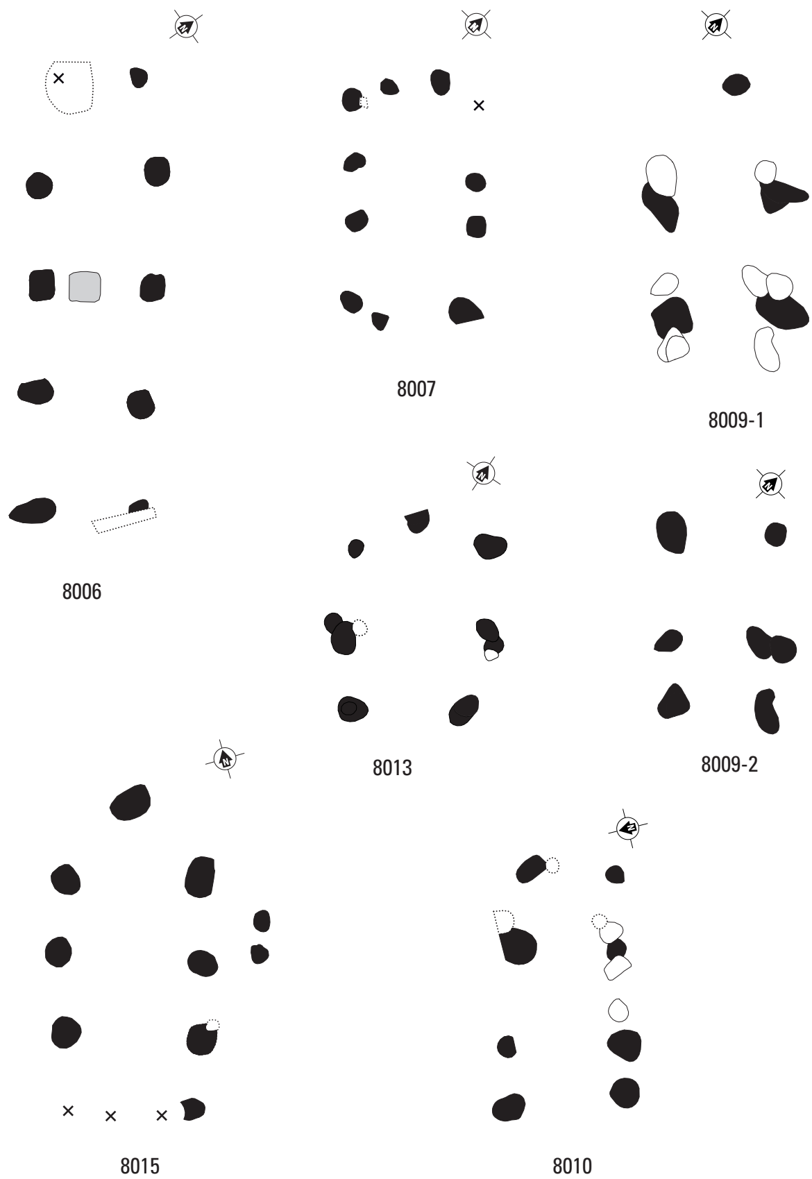
Fig. 5.23. Wijchen-Oostflank. Overzicht van de volmiddeleeuwse huisplattegronden op de Oostflank.
