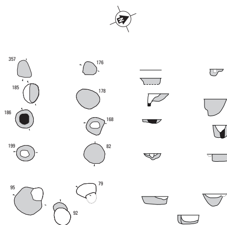
Fig. 17.19. Wijchen-Oostflank. Plattegrond van huis 8012. Schaal 1:200. NAP 8.60.
