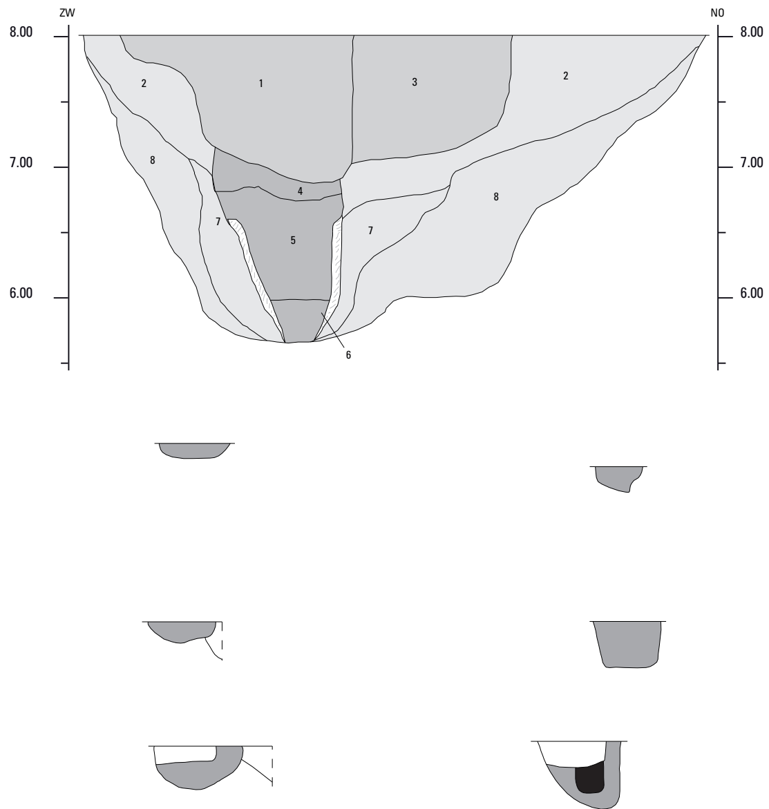
Fig. 17.30B. Wijchen-Oostflank. Waterput 7005, Schaal 1:40.
