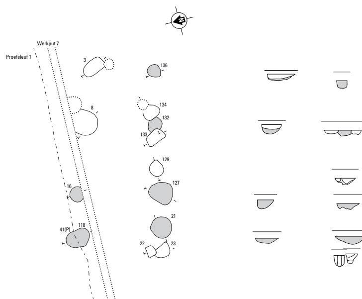
Fig. 17.18. Wijchen-Oostflank. Plattegrond van huis 8010. Schaal 1:200. NAP 8.20.
