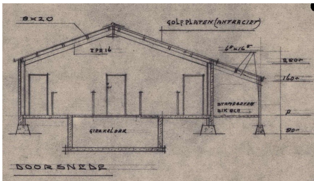
Figuur 38: Dwarsdoorsnede bouwtekening uit 1975 (gemeentearchief Wijchen).
